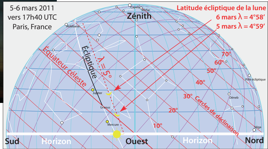
▼ Fig. 2b. Solarium : lune en berceau les 5 et 6 mars 2011. Cliché : Comité de liaison enseignants-astronomes (reprise DAO : A. Dumontet et C. Touzel, ARTeHIS).
