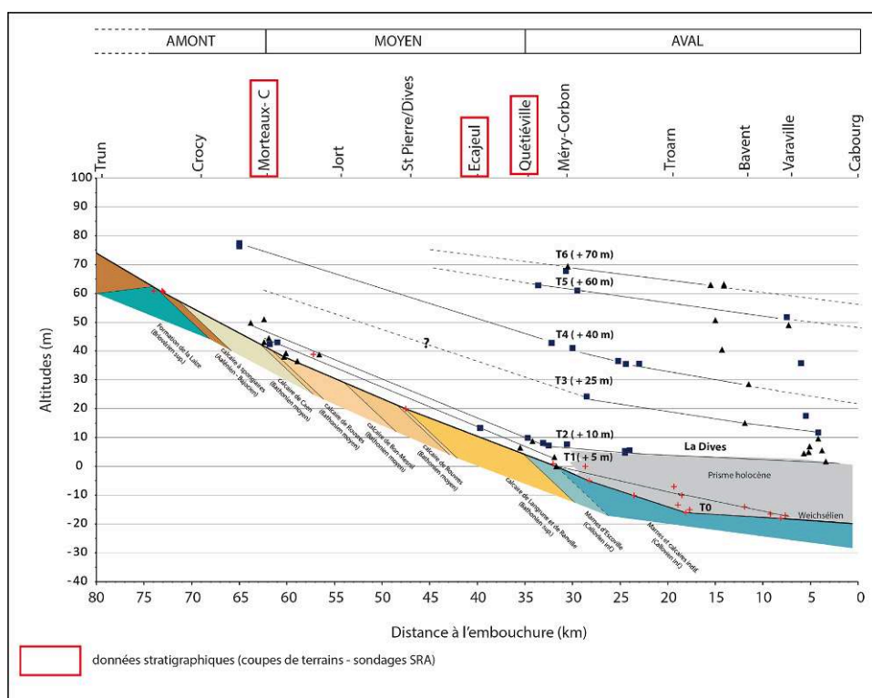
Fig. 1 – Profils longitudinaux de la dernière incision et terrasses alluviales de la Dives
