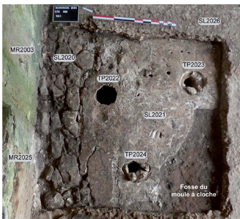
Fig. 2 – Relevé en plan des divers sols en lien avec l'église et des structures en creux qui percent SL2021 (avant leur fouille)
