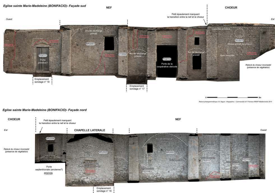
Fig. 1 – Relevé photogrammétrique des façades sud et nord
