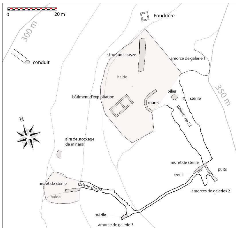
Fig. 1 – PLAN DES STRUCTURES MINIÈRES DE RENINCA : SITES 23 ET 24
