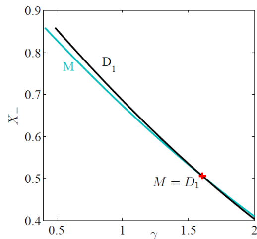
図2：2目的パラメータ探索。 X_- は制御しきい値、 \gamma は制御クロックに対応するパラメータ。カーブ D_1 は安定境界、カーブ M は最大電力点に対応。その交点(赤)が目標値。
