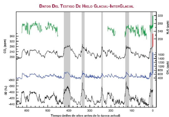
Figura 6.3. Glaciaciones e interglaciaciones (IPCC.07). Variaciones del deuterio D en el hielo ártico representativo de la temperatura local y variaciones de las concentraciones de CO_2 , CH_4 y N_2O . Barras grises: interglaciaciones.
