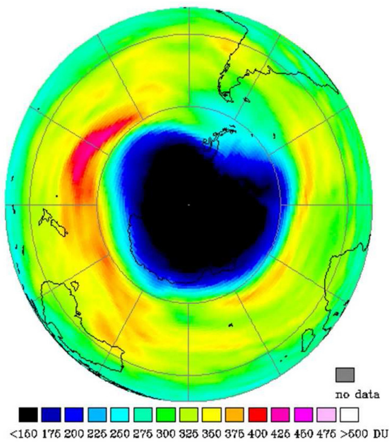
Figura 5.6. Mapa de la columna de ozono sobre la región austral durante la fase de apogeo del agujero de ozono. Los valores en el interior del vórtice antártico oscilan entre 100 y 150 DU (Datos OMS/NASA).
