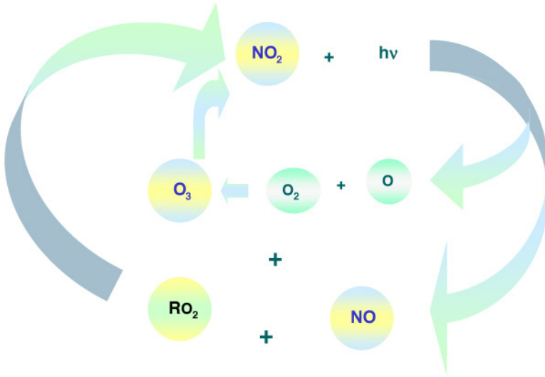
Figura 3.3. Ciclo de formación de ozono en atmósfera contaminada.
