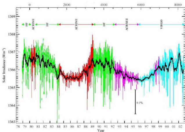
Figura 2.2. Variabilidad de la Constante Solar ( \text{W/m}^2 ) desde 1978 hasta 2003. En la parte superior de la gráfica son indicados los diferentes satélites utilizados para su determinación. (Fuente: www.gsfc.nasa.gov/topstory/2003/0313irradiance.html ).
