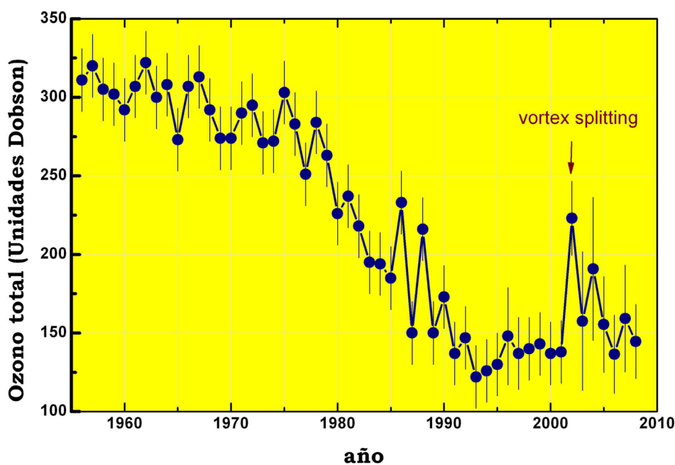
Figura 5.9. Evolución del ozono en la Antártida desde el comienzo de las medidas (fuente: BAS). Valores medios para octubre de la columna de ozono medidos en la base británica de Halley Bay.
