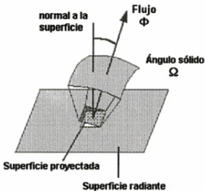
Figura 2.4. Interpretación geométrica de la radiancia (Sobrino et al., 2000).
