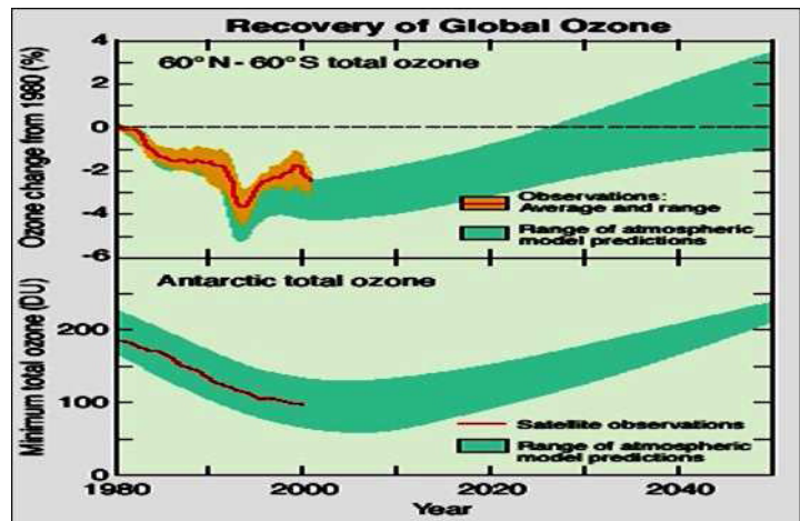
Figura 5.12. Evolución de la anomalía del ozono global (medias planetarias) con el tiempo. Las predicciones futuras presentan mucha incertidumbre como ponen de manifiesto las estimaciones basadas en modelos (Fuente OzoneAssessment, WMO 2003).
