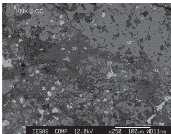
写真1 世羅町採取鉱石 (KNK-1) の反射電子像
