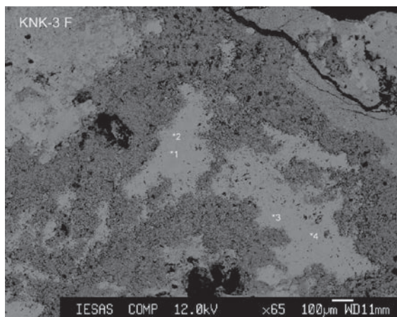
写真2 カナクロ谷遺跡出土鉱石 (KNK-3) の反射電子像
