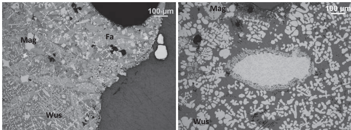
写真3 カナクログ谷出土鉄滓 (左：KNK-6 右：KNK-7)
