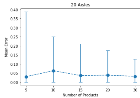
(d) Error trend for 20 aisles
