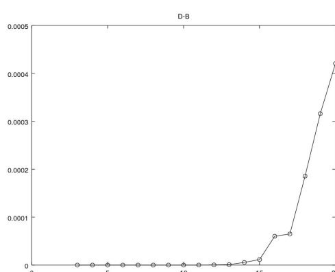
Slika 2.5: \|X_l - X_3\|
