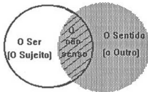
Figura 4 – Alienação em referência aos conjuntos do Ser e do Sentido.
