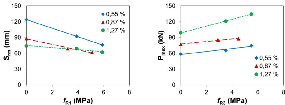
Figura 6: Efecto de la resistencia residual sobre diferentes parámetros medidos en vigas de hormigón armado: espaciamento medio de fisuras (izq) carga máxima (der.)
