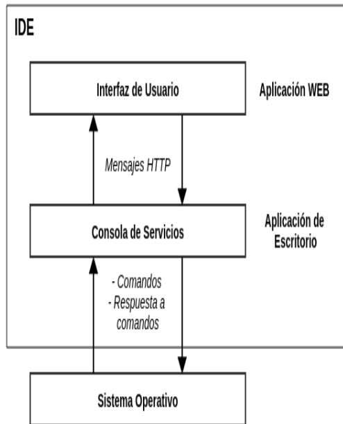
Fig. 3 Detalles de implementación del IDE
