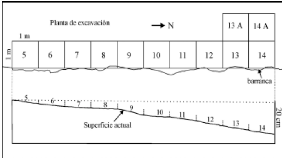
Figura 6.45. Planta de excavación y corte transversal del buzamiento de barranca
