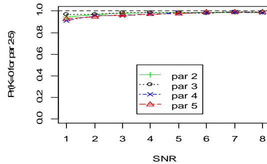
Fig 2d - Par 2-5: True K = 0
