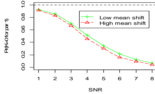
Fig 2f - Par 1: True K = 1, True Q = 9
