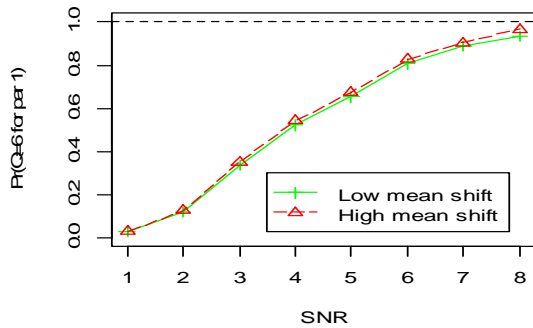
Fig 2c - Par 1: True K = 1, True Q = 6
