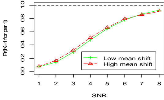
Fig 2e - Par 1: True K = 1, True Q = 9
