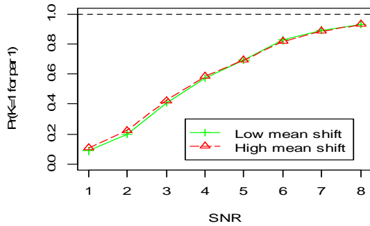
Fig 2a - Par 1: True K = 1, True Q = 6
