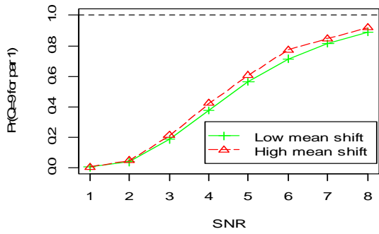
Fig 2g - Par 1: True K = 1, True Q = 9
