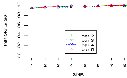
Fig 2h - Par 2-5: True K = 0
