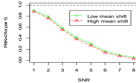
Fig 2b - Par 1: True K = 1, True Q = 6
