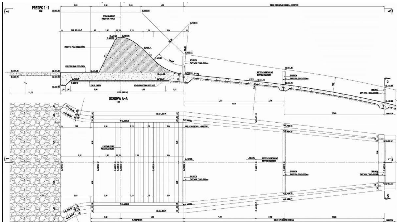
Слика 8. Чеони прелив – основа и пресек
