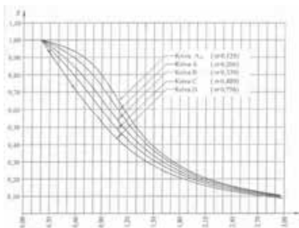
Slika 8. Krive izvijanja prema našim propisima (preuzeto iz [3]) Figure 8. Buckling curves according to JUS (taken from [3])
