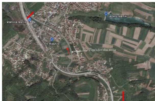
Slika 13. Deo sliva Topčiderske reke sa granicama računске deonice [12].
