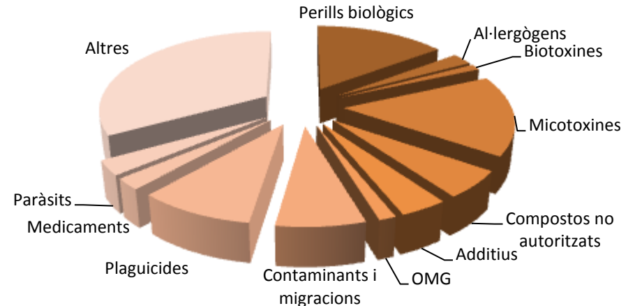
Alertes gestionades a Catalunya segons dades de l'ASPCAT. Distribució proporcional de les 78 alertes registrades el 2011
