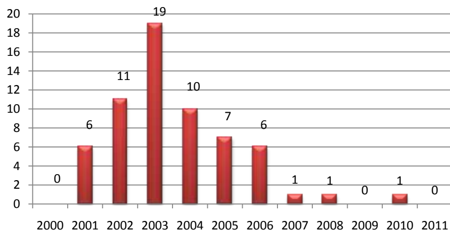
Nombre de casos confirmats d'encefalopatia espongiforme bovina (EEB) segons dades del DAAM. Catalunya 2000 - 2011
