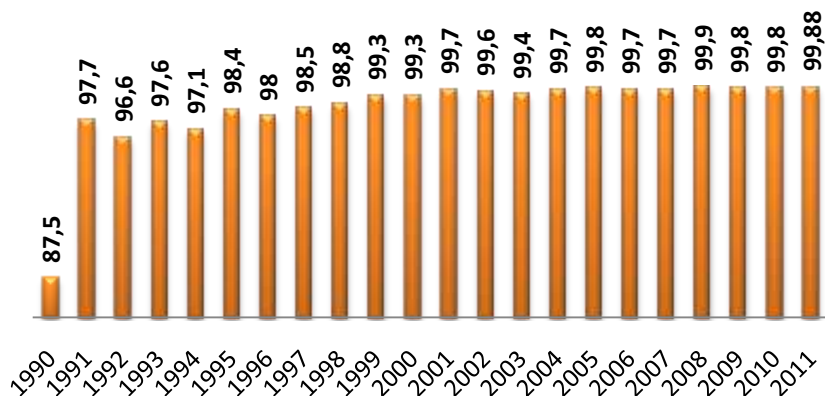
Evolució de resultats del Pla d'investigació de residus en aliments d'origen animal segons dades de l'ASPCAT. Taxes de conformitat (%). Catalunya 1990-2011
