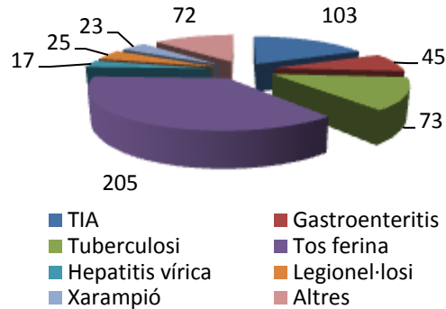
Nombre de brots de TIA comparats amb altres tipus de brots declarats. Catalunya 2011
