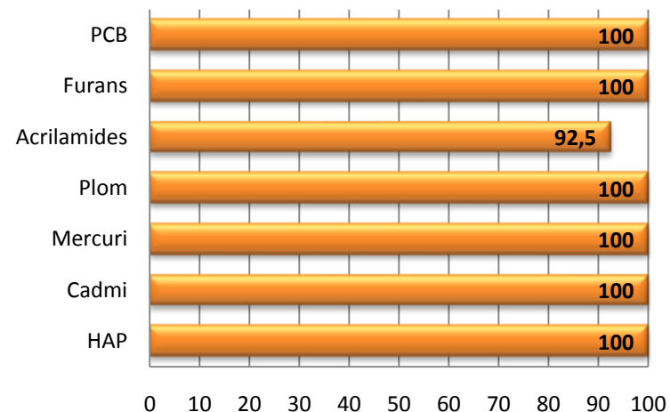
Taxes de conformitat per a contaminants determinats segons dades de l'ASPB (%). Catalunya 2011
