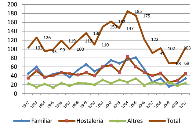
Nombre de brots de malalties de transmissió alimentària notificats. Catalunya 1992-2011
