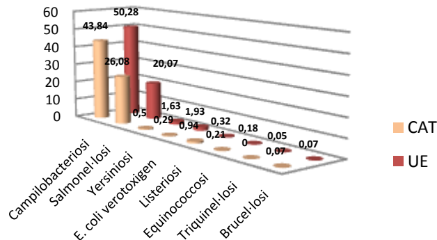
Comparativa de notificació per 100.000 habitants de les principals malalties de transmissió alimentària. Catalunya (CAT)–mitjana Unió Europea (UE) 2011 (2)
