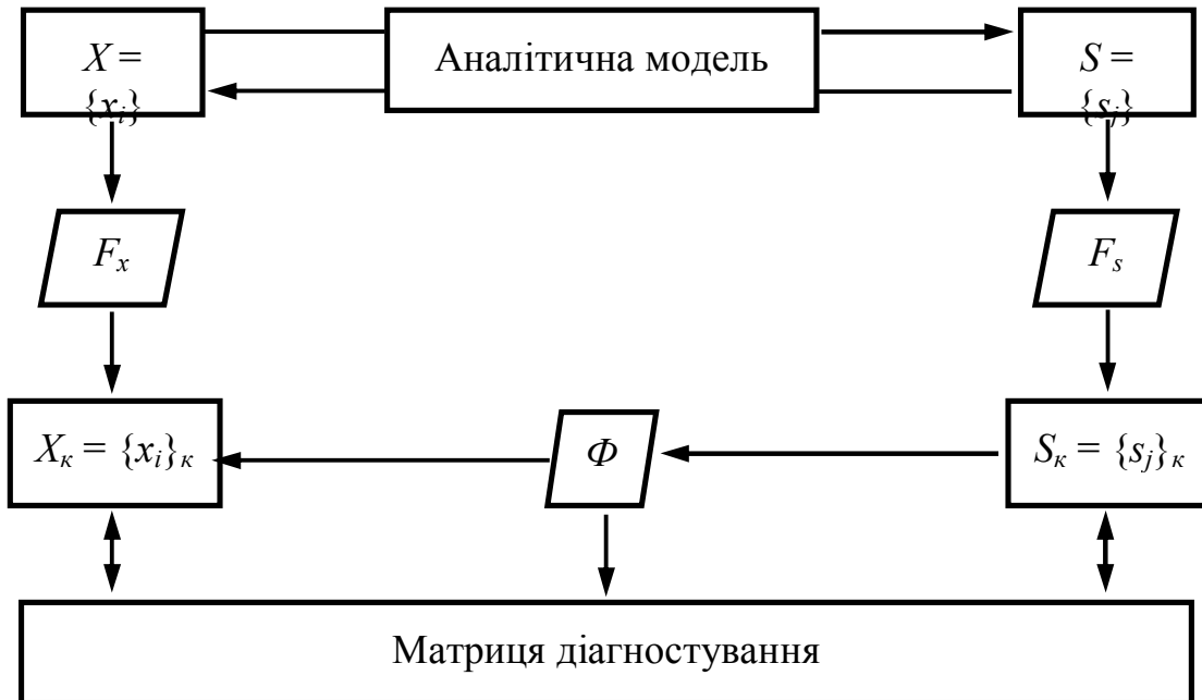
Рис 2. Блок-схема синтезу матриці діагностування: X = \{x_{ij}\} – нескінченна кількість технічних станів об'єкта; X_k = \{x_{ij}_k\} – кінцева кількість технічних станів; S = \{s_{ij}\} – нескінченна множина ознак технічних станів об'єкта;
