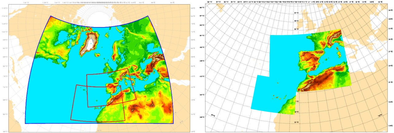
Figura 20.11: Dominios de integración de los modelos integrados en AEMET: HIRLAM a la izquierda, HARMONIE-AROME a la derecha. (ampliación en Figura 20.12 en la página siguiente). AEMET.
