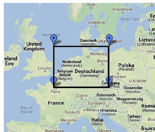
Figura 20.6: Calibración del viento a 10 m. Realizando el entrenamiento en áreas relativamente pequeñas, los resultados para umbrales altos pueden mejorar (ver texto). FROGNER, 2014.
