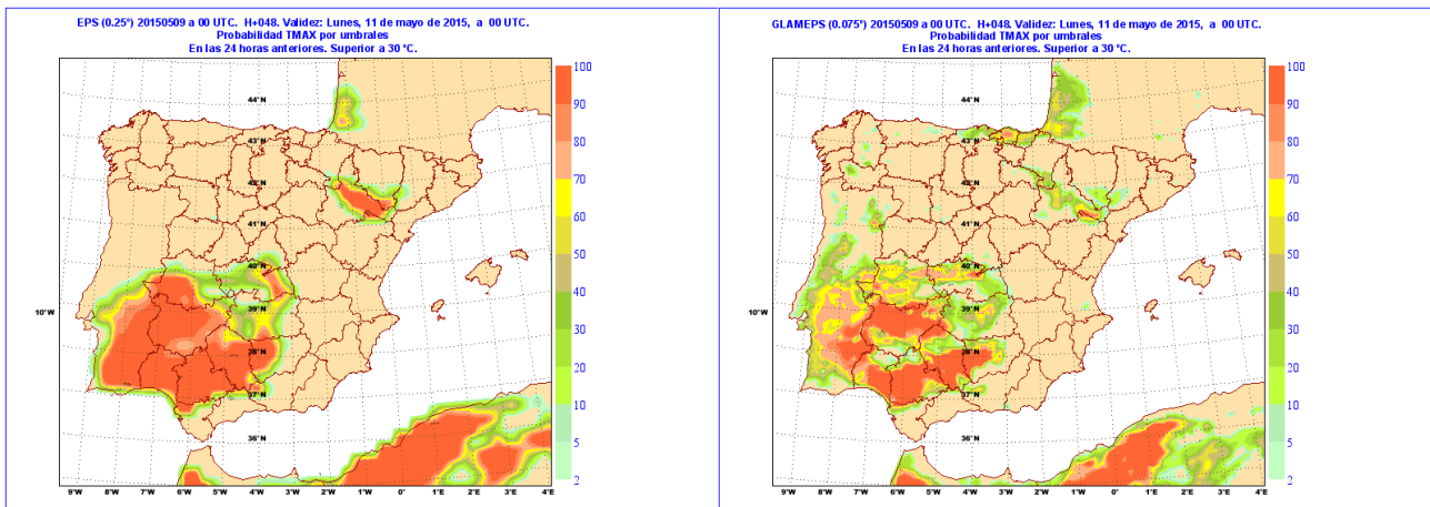
Figura 20.8: Probabilidad de temperaturas por encima de 30 °C como herramienta de decisión para emisión de avisos. A la izquierda ECENS con resolución horizontal de 16 km. A la derecha GLAMEPS con 7.5 km. La capacidad de GLAMEPS para afinar por pequeñas regiones es notable (ver texto).
