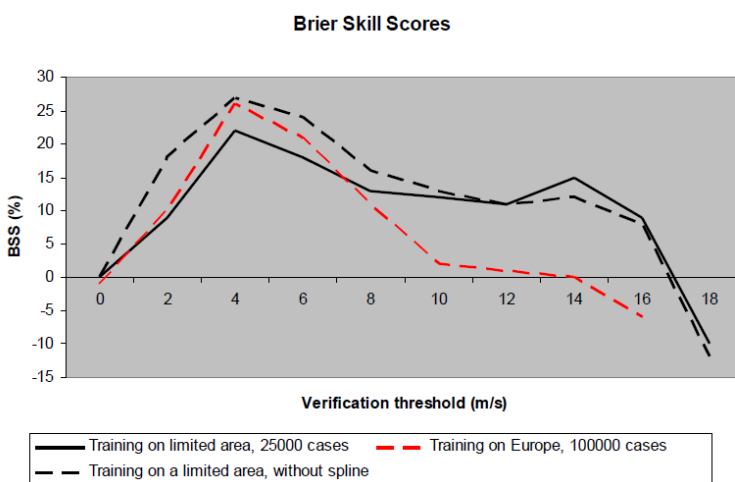
Figura 20.6: Calibración del viento a 10 m. Realizando el entrenamiento en áreas relativamente pequeñas, los resultados para umbrales altos pueden mejorar (ver texto). FROGNER, 2014.
