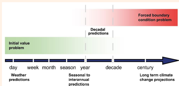
Figura 29.16: Esquema que ilustra la progresión desde las predicciones a escalas temporales cortas, que constituyen un problema de valores iniciales, a las proyecciones climáticas, que son problemas de condiciones de contorno forzadas. La predicción decadal ocupa el término medio entre ambos (Fig. 1.2 de Kirtman et al. 2013 [23]).
