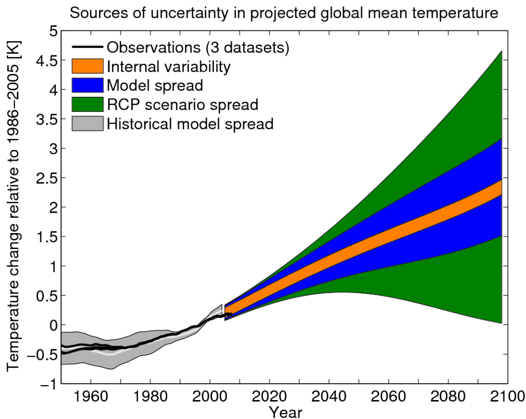
Figura 29.1: Fuentes de incertidumbre en la simulación climática (fuente: Cubasch et al. 2013 [8]).
