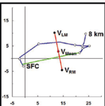
Figura 3: Storm-splitting como se observaría en una imagen radar (figura de arriba) y valores del vector movimiento de las células divididas (a derecha e izquierda del viento medio) representados sobre una hodógrafa (figura de la izquierda). La línea verde indica el vector cizalladura. Los vectores movimiento de cada célula se sitúan 7.5 \text{ m/s} a izquierda y derecha del viento medio de los 6 km junto al suelo, sobre una perpendicular al vector cizalladura. Fuente: The Comet Program y elaboración propia.
