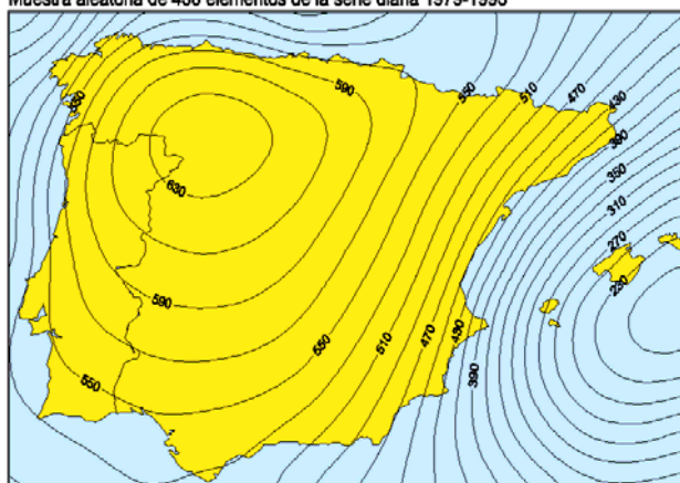
Mapa de Correlación para TM 12h en Oviedo con 25 Análogos Predictor: TSup 12z Serie ECMWF Re-Análisis Muestra aleatoria de 430 elementos de la serie diaria 1979-1993
