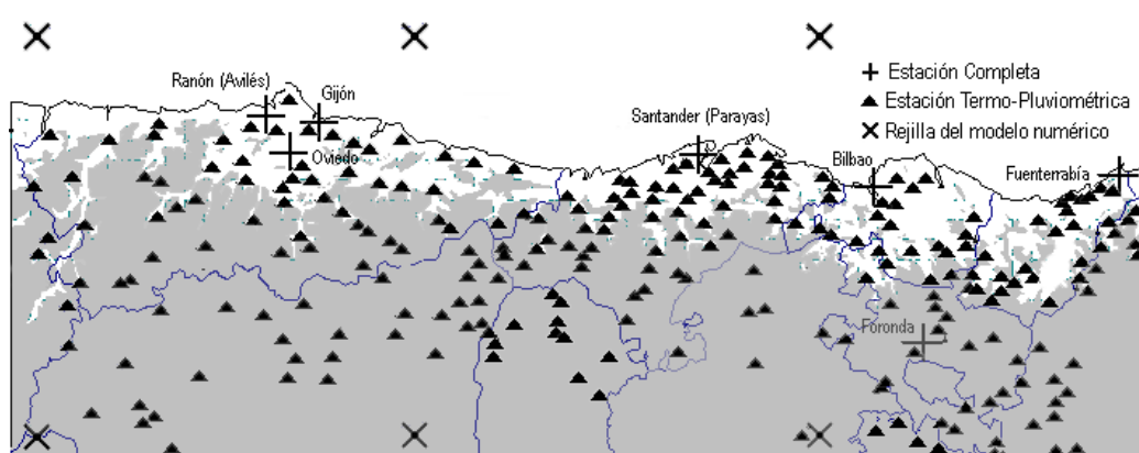
Figura 1. Estaciones completas (+) y termo-pluviómetricas (▲) de la Red Nacional de Observatorios del I.N.M. del Centro Meteorológico Territorial de Cantabria y Asturias. También se muestran los correspondientes puntos de rejilla (X) del modelo climático del Centro Hadley.
