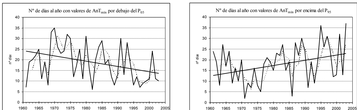
Fig. 3. Evolución temporal de la frecuencia anual de días con anomalías de temperatura mínima por debajo del umbral definido por el P_{05} , y por encima del umbral definido por el P_{95} en el intervalo 1961-2003.
