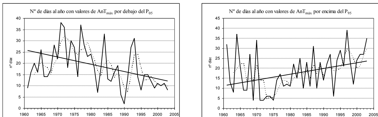
Fig. 2. Evolución temporal de la frecuencia anual de días con anomalías de temperatura máxima por debajo del umbral definido por el P_{05} , y por encima del umbral definido por el P_{95} en el intervalo 1961-2003.
