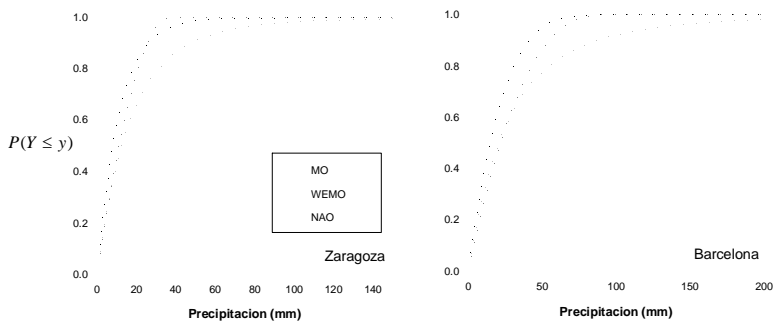
Fig. 4. Curvas de probabilidad de no excedencia correspondientes a la máxima intensidad de precipitación diaria en los eventos positivos y negativos de la NAO, WeMO y MO en los observatorios de Zaragoza y Barcelona. Línea discontinua: eventos negativos. Línea continua: eventos positivos.
