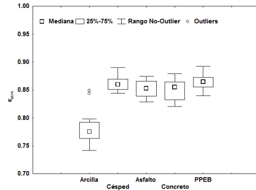
Fig. 3: Variabilidad de la \epsilon_{atm} en las superficies estudiadas
