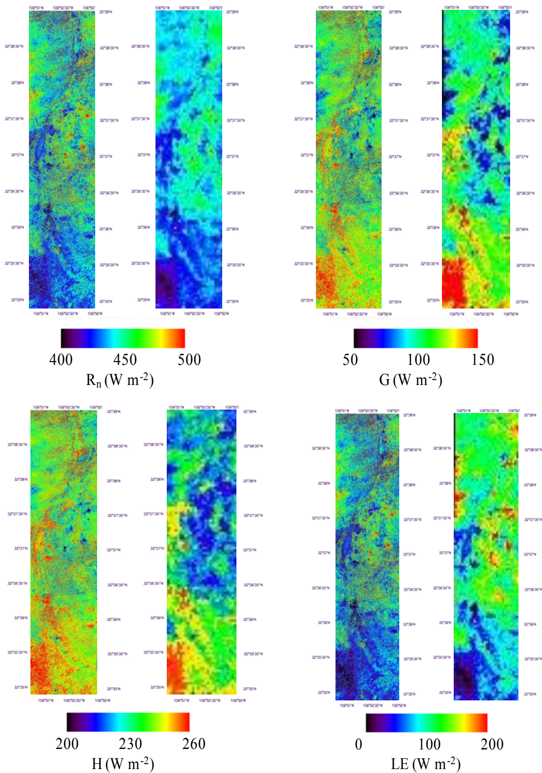
Fig.3: Mapas de flujos energéticos sobre Jornada para el día 20/5/2004 (11:36 GMT). Vuelo MASTER con píxeles de 3 m (izquierda); simulación HypSPIRI con píxeles de 60 m (derecha).
