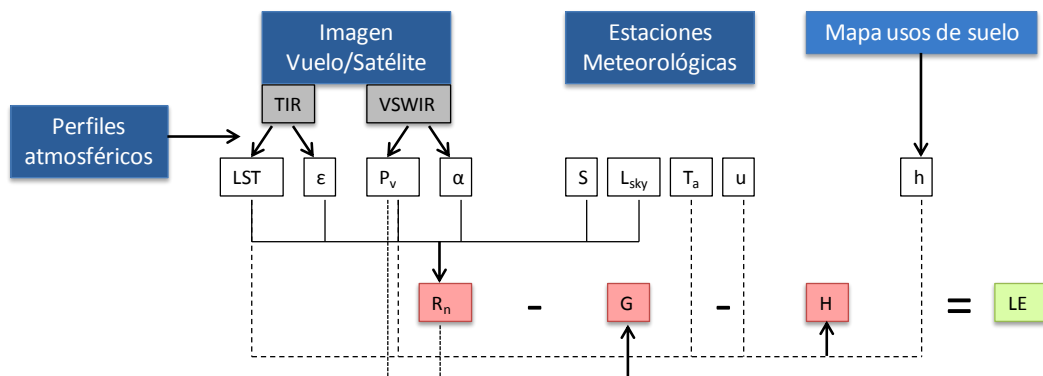
Fig. 2: Esquema del modelo simplificado de dos fuentes STSEB.
