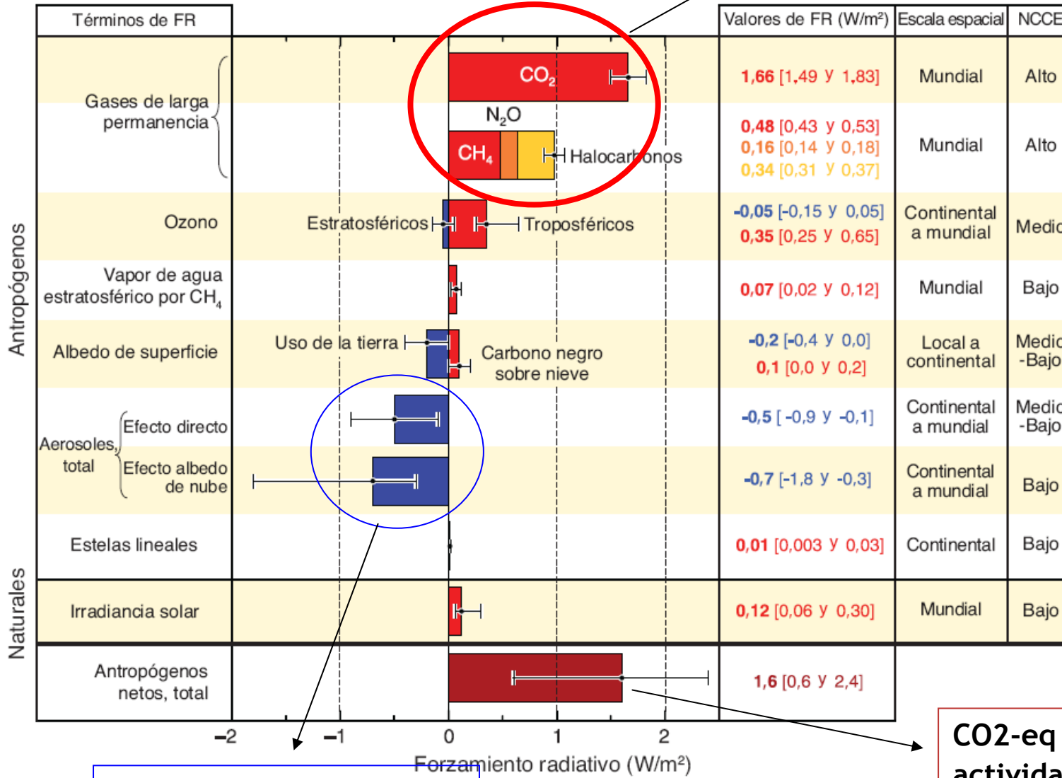
Componentes del forzamiento radiativo
