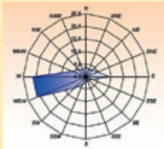
Figura 8. Rosas de viento estacionales elaboradas con los datos de la estación de Caravaca "Fuentes del Marqués", período 2009-2016.
