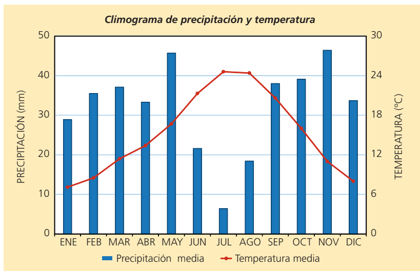
Figura 4. Precipitación media mensual (columnas azules) y temperatura media mensual (línea roja) del periodo de referencia 1981-2010.
