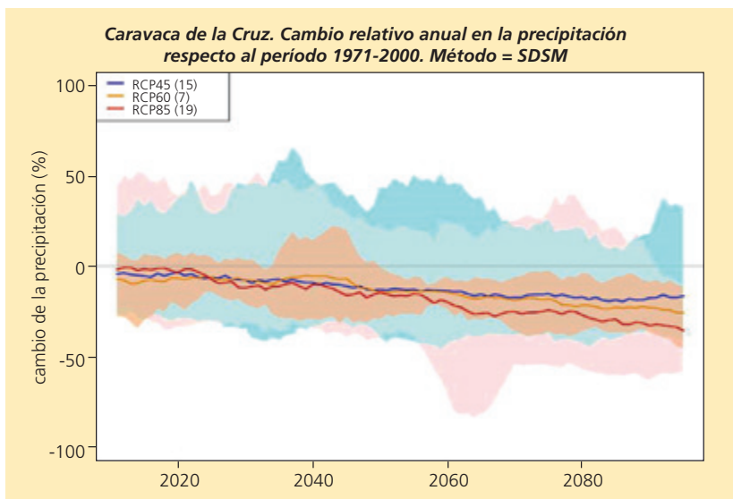
Figura 11. Las líneas continuas representan la proyección media del conjunto de modelos para cada uno de los tres escenarios de forzamiento empleados.
