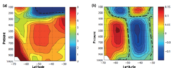
Figura 3: Climatología (a) y primer modo de variabilidad (b) de la baroclinicidad promediada zonalmente en el HS.
