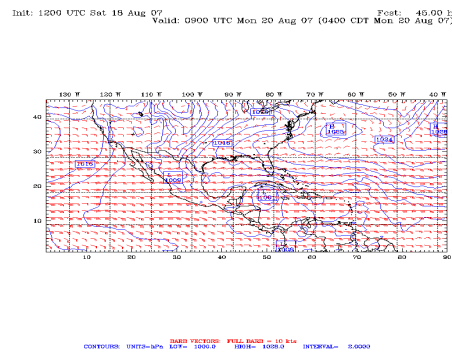
Fig. 5 Mapas del tiempo del Estado de Jalisco (a) y de la República Mexicana (b) obtenidos del modelo WRF
