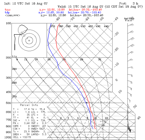
Fig. 6 Sondeos atmosféricos derivados del modelo de análisis y pronóstico del tiempo WRF para la ZMG.
