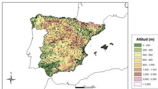
Fig. 2.- Distribución espacial de las observaciones pluviométricas el 31 de diciembre de 2004
