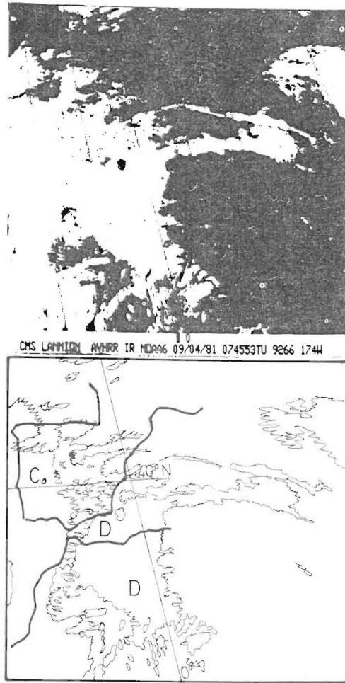
Fig. 37.- Imagen satelitaria (IR) recibida del NOAA 6 (parte superior). Esquema de los sistemas nubosos y referencias geográficas (parte inferior). 9 de abril de 1981 a las 0745TMG.
