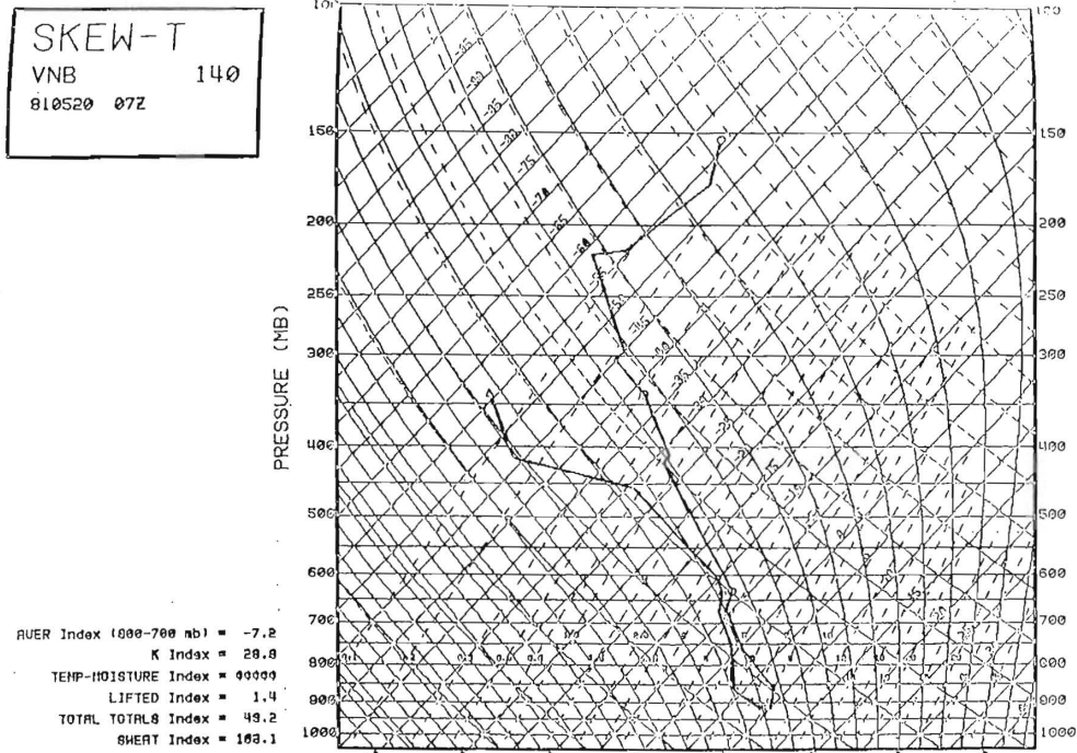
Fig. 6.- Sondeo aerológico en Villanubla de las 0700TMG
