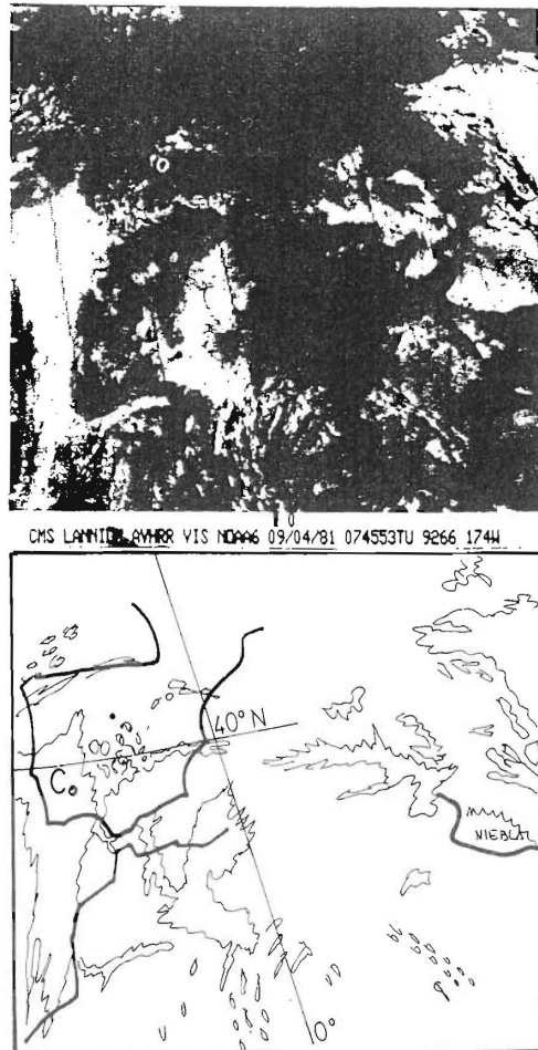
Fig. 36.- Imagen satelitaria (VIS) recibida del NOAA 6 (parte superior). Esquema de los sistemas nubosos y referencias geográficas (parte inferior). 9 de abril de 1981 a las 0745TMG.
