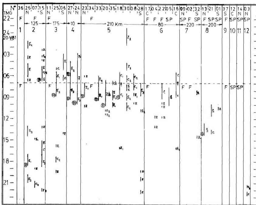
Fig. 14.- Diagrama de franjas (DF). Ver el texto para la explicación de los símbolos usados.
