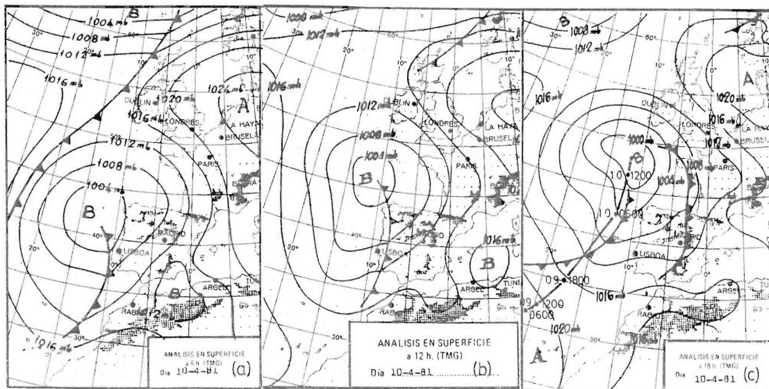
Fig. 20.- Mapas sinópticos de superficie (Boletín del I.N.M.) para el 10 de abril de 1981.
