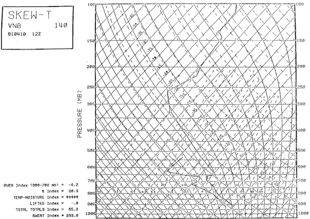
Fig. 27.- Sondeo aerológico en Villanubla el día 10 de abril de 1981 a las 1200Z.
