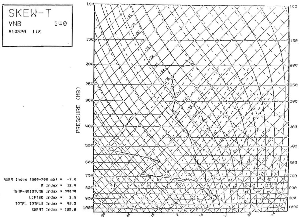
Fig. 7.- Sondeo aerológico en Villanubla de las 1100TMG
