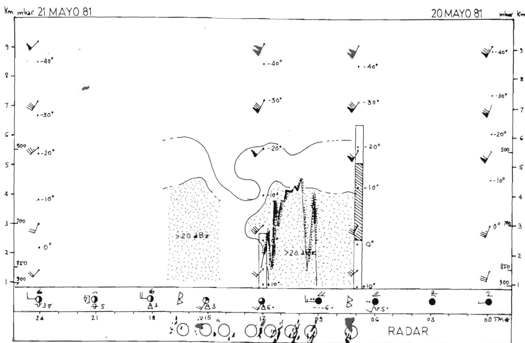
Fig. 12.- Corte transversal de la atmósfera sobre Villanubla (20 de mayo de 1981). Ver el texto para la explicación de los símbolos usados.
