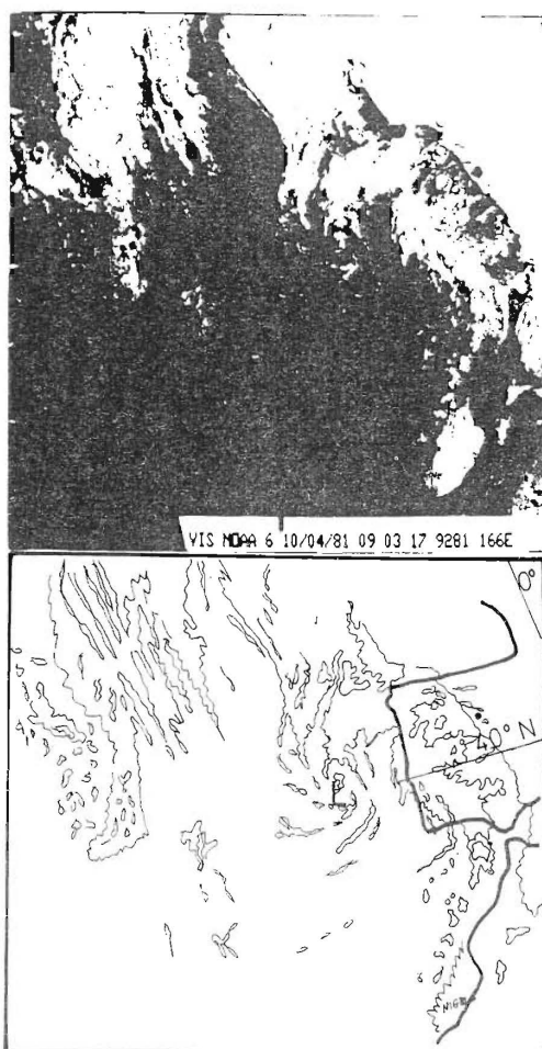
Fig. 39.- Imagen satelitaria (VIS) recibida del NOAA 6 (parte superior). Esquema de los sistemas nubosos y referencias geográficas (parte inferior). 10 de abril de 1981 0903Tmg.
