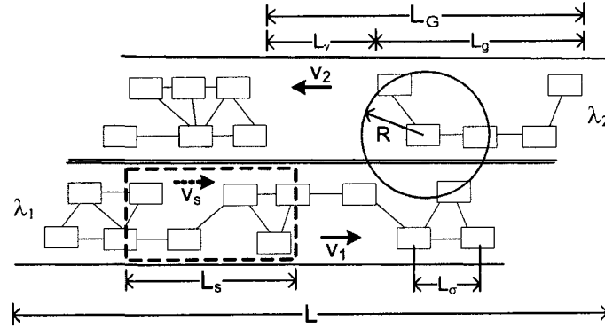
Fig. 24: HOG Variables.
