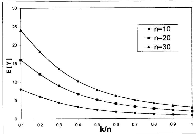
FIG. 26: E[Y] vs. k/n
