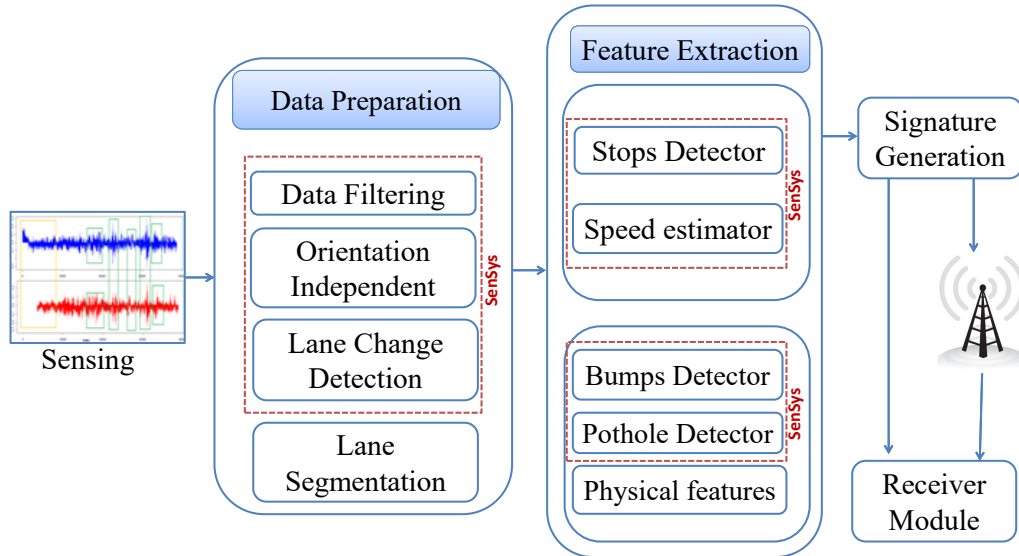
FIG. 45: inLaneCom Framework
