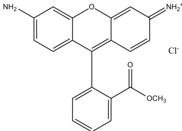
Rhodamine 123
