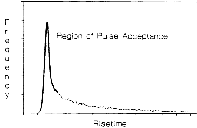
Fig. 2 CdTe pulse risetime spectrum
