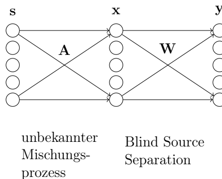
Abbildung 3.5: Feedforward Netz des InfoMax Algorithmus
