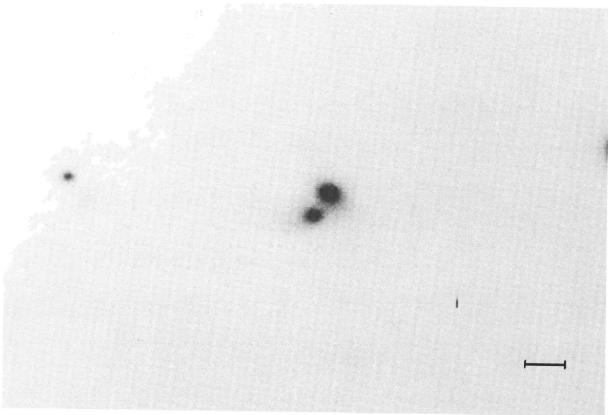
FIG. 3.—IRAS 08572+3915
