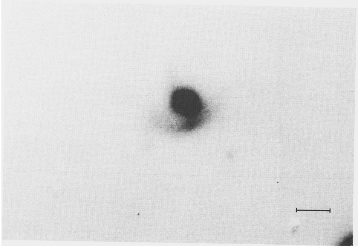
FIG. 5.—IRAS 12112+0305
