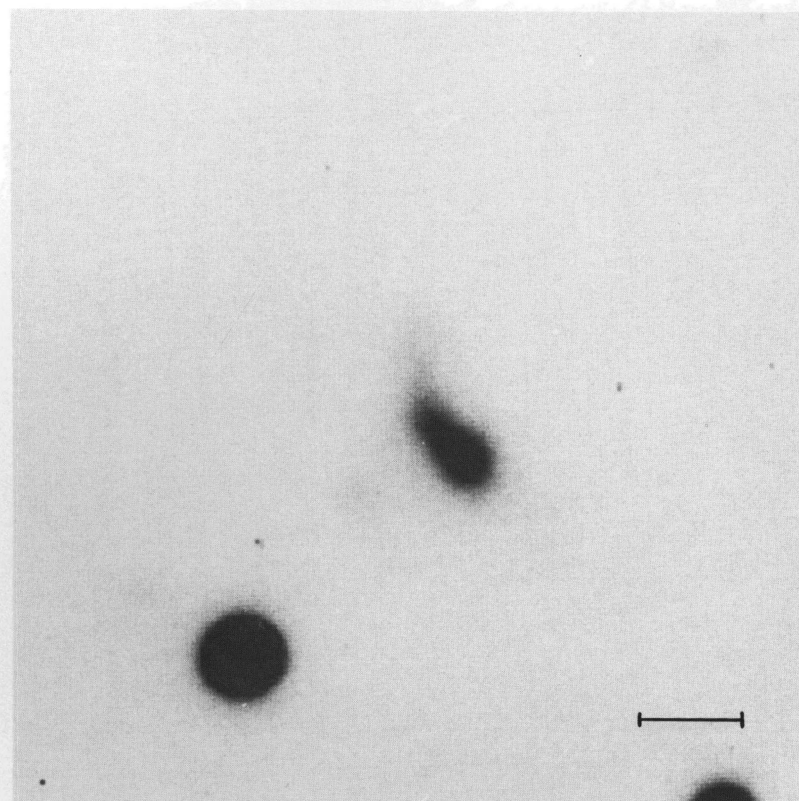
FIG. 8.—IRAS 14348—1447
