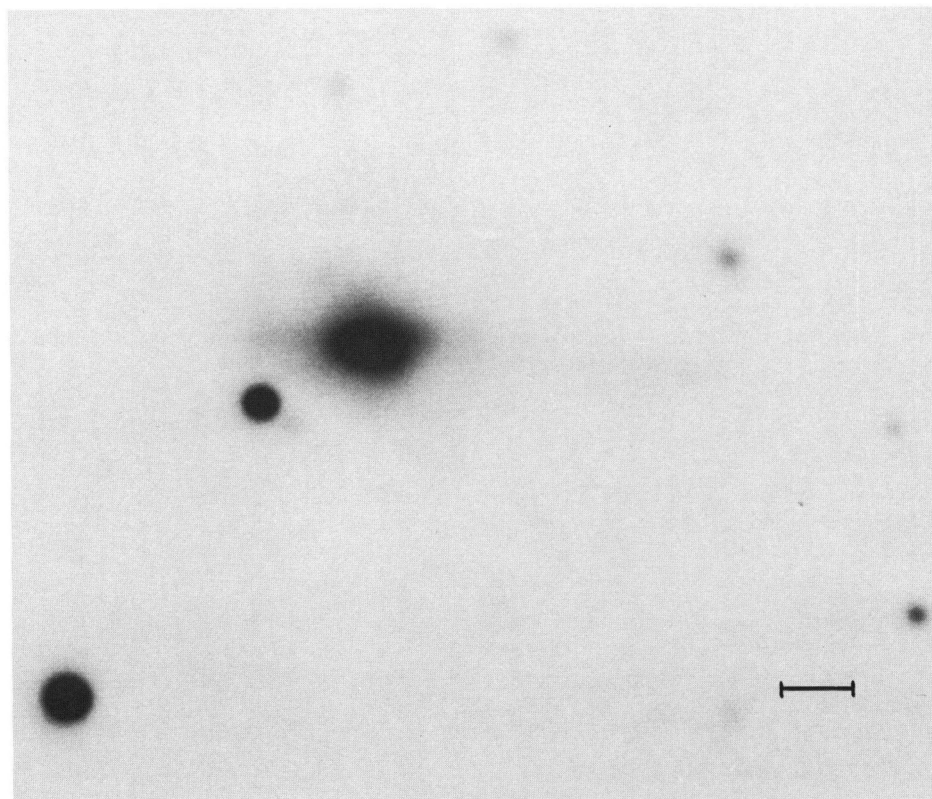
FIG. 4.— IRAS 09320+6134 = UGC 05101
