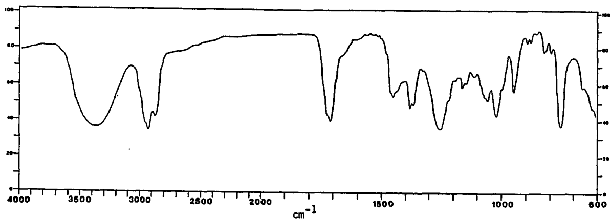
IR Spectrum of 121
