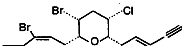
8 isodactylyne
