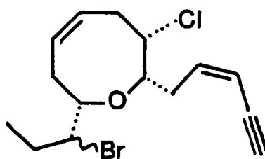
10 cis-isodihydrorhodophytin
