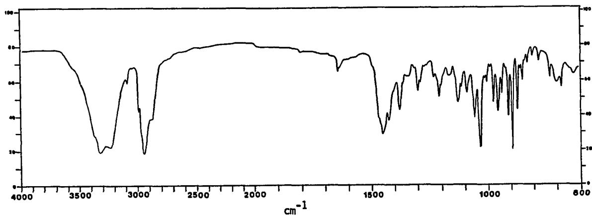
IR Spectrum of 124
