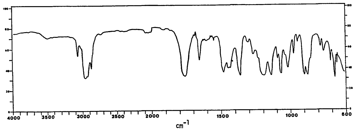
IR Spectrum of 101
