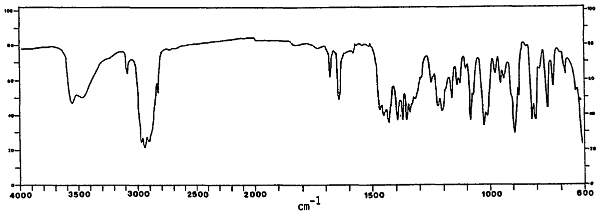
IR Spectrum of 100
