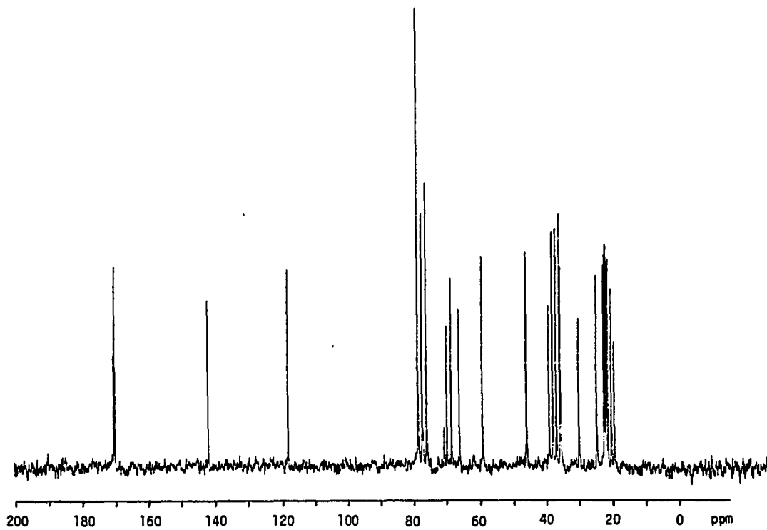
25.05 MHz ^{13}\text{C} -NMR ( \text{CDCl}_3 ) Spectrum of Parguerol ( 110a ).
