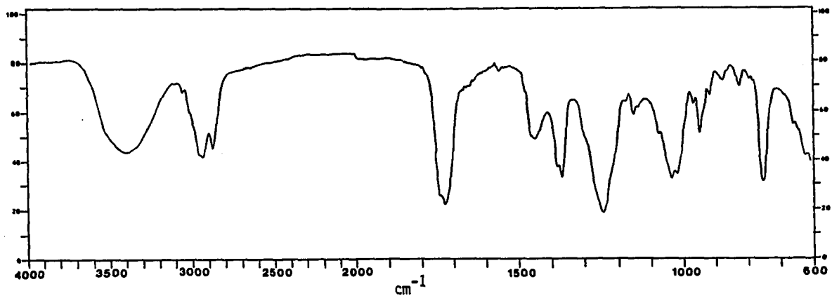
IR Spectrum of 118
