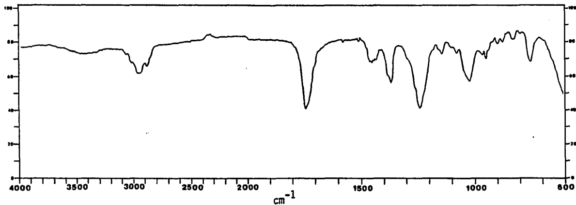
IR Spectrum of 110a
