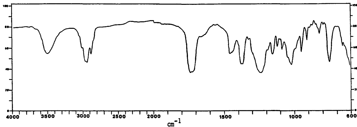
IR Spectrum of 122
