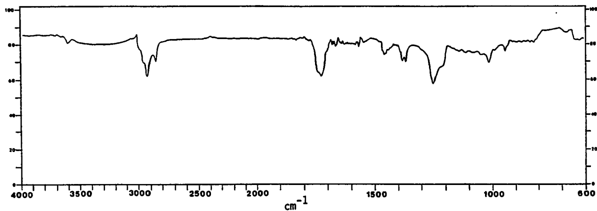
IR Spectrum of 123
