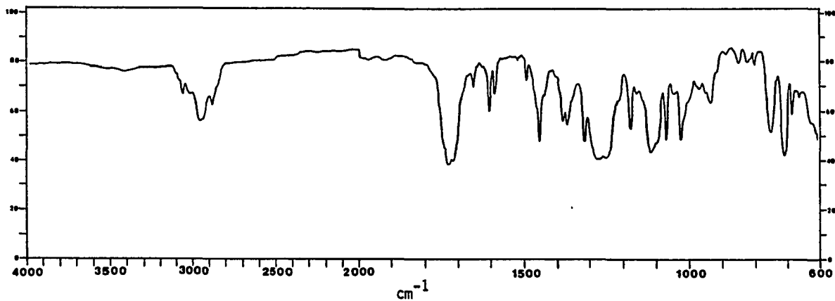
IR Spectrum of 110b
