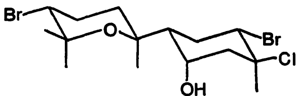
31 deodactol
