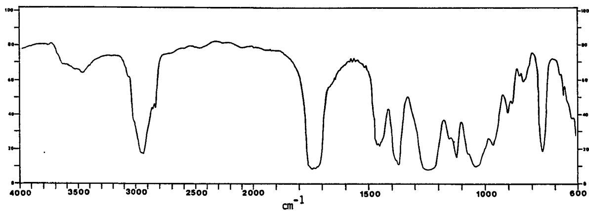
IR Spectrum of 111
