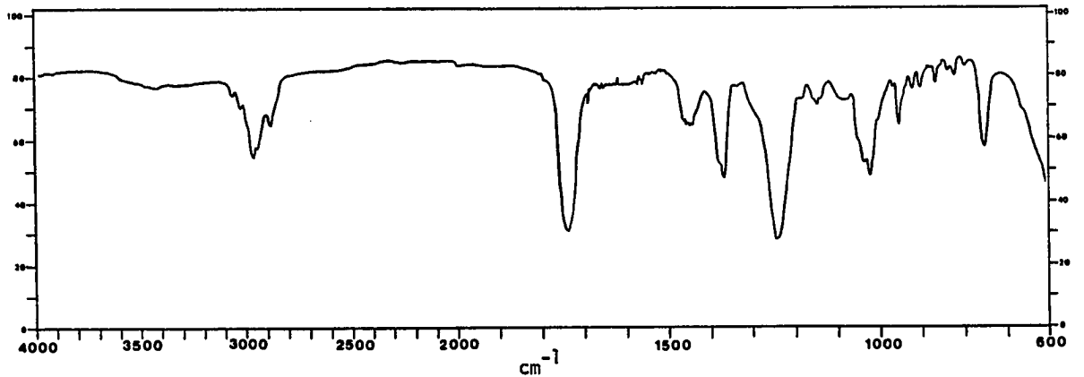
IR Spectrum of 120
