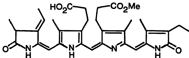
91 alysiaverdin
