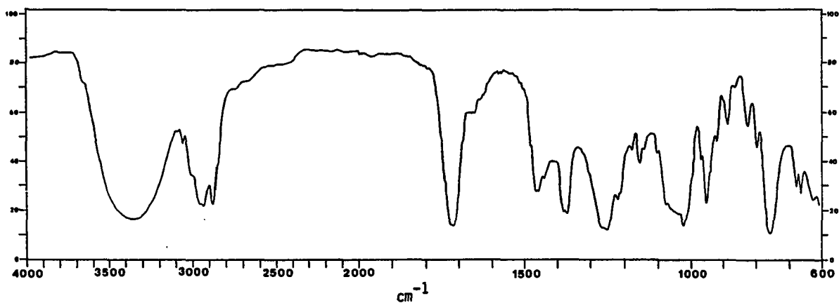
IR Spectrum of 109
