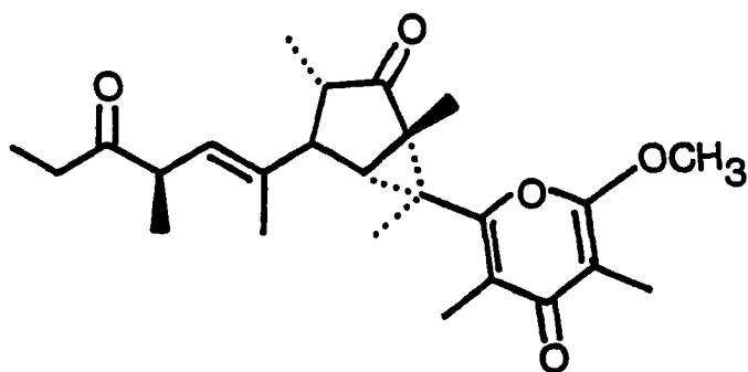
74 crispatone
