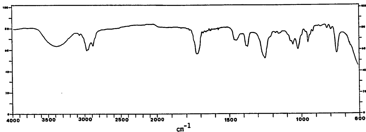
IR Spectrum of 119
