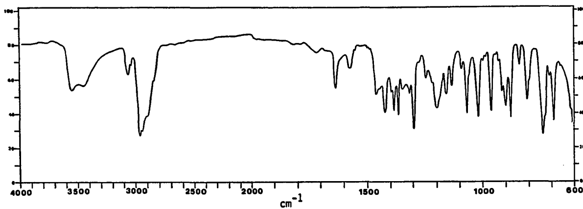
IR Spectrum of 104a
