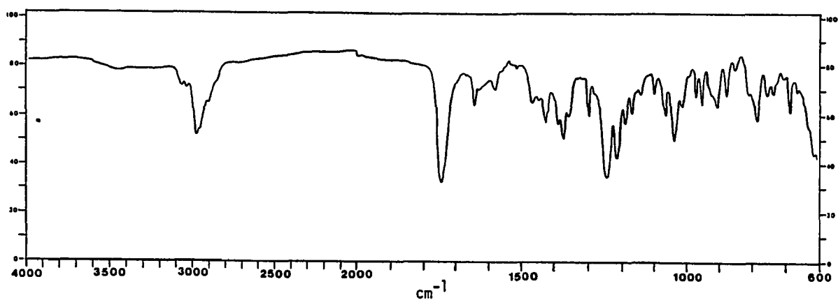
IR Spectrum of 105b
