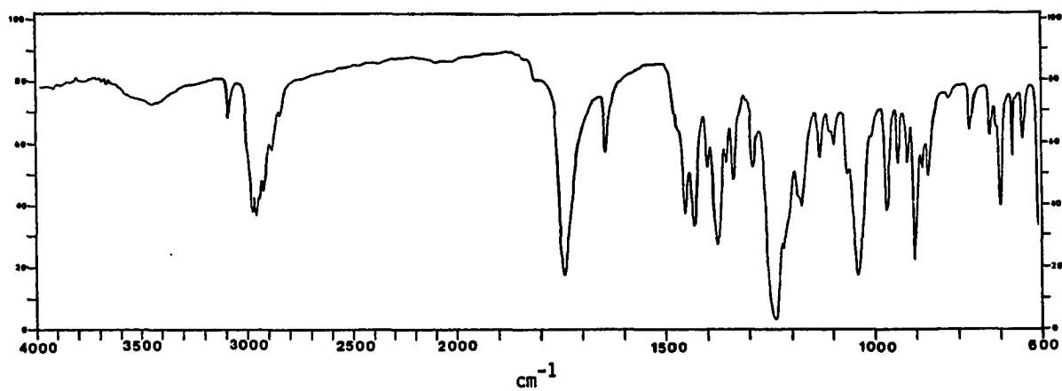
IR Spectrum of 108
