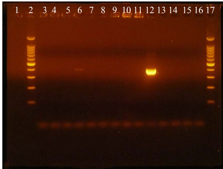
Figure 19: Specificity of primer set HE1/HE3 nested. 2% agarose gel run for 1hour 10min at 100V. Lanes: 1) blank, 2) 100bp DNA ladder, 3) A. americanum adult, 4) A. americanum nymph, 5) D. variabilis adult, 6) D. variabilis nymph, 7) I. scapularis adult, 8) I. scapularis nymph, 9) A. phagocytophilum , 10) A. odocoilei , 11) B. burgdorferi , 12) E. chaffeensis , 13) F. tularensis , 14) R. rickettsii , 15) negative, 16) 100bp DNA ladder, 17) blank.
