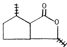
C-1 3a
