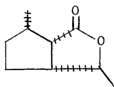
C-3 3c
