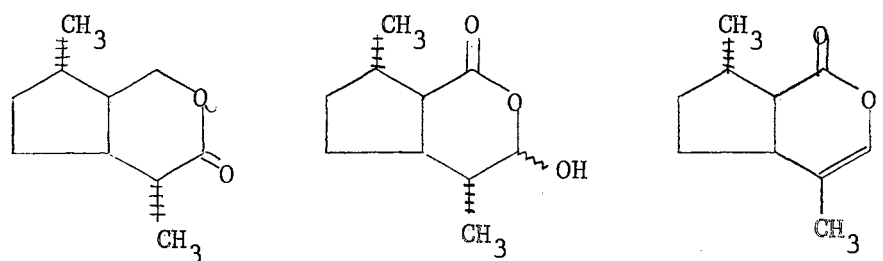
Isoiridomyrmecin
