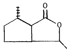
C-2 3b
