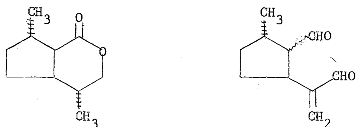
Isodihydro- nepetalactone
