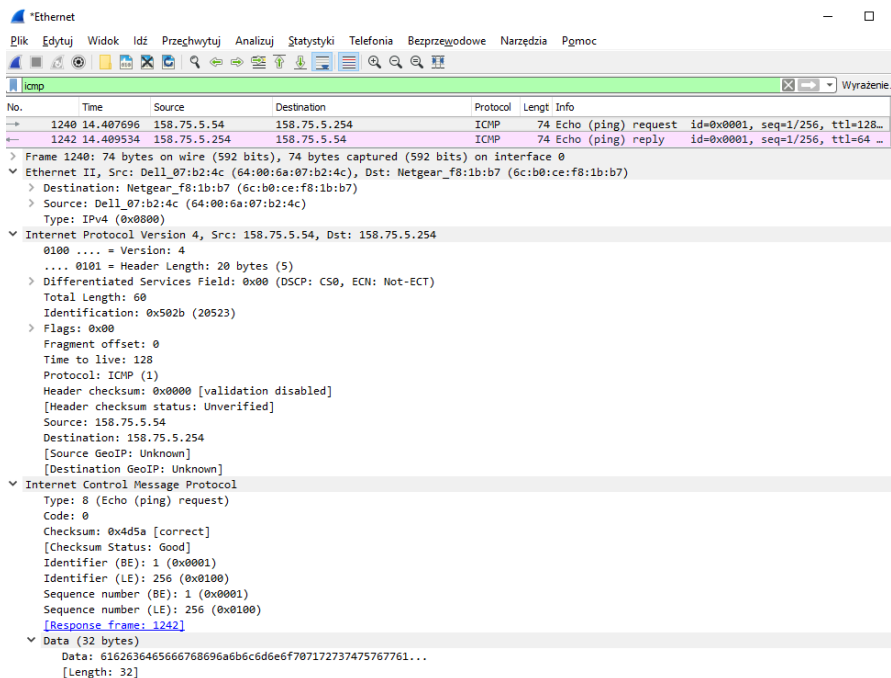
Rysunek 2 Dane przechwycone w programie Wireshark związane z testem osiągalności interfejsu bramy domyślnej.
