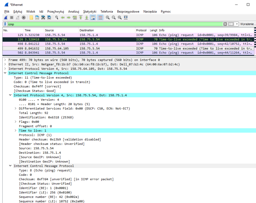
Rysunek 4 Dane przechwycone w programie Wireshark związane z testem śledzenia ścieżki do zdalnego hosta za pomocą komendy tracert.
