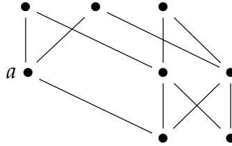
Rysunek 2.2: Diagram Hassego ściągającej, skończonej przestrzeni topologicznej X z punktem wyróżnionym a o tej własności, że (X, \{a\}) jest \mathcal{C} -rdzeniem, a zatem przestrzeń X nie jest \mathcal{C} -rozbiegalna do a .
