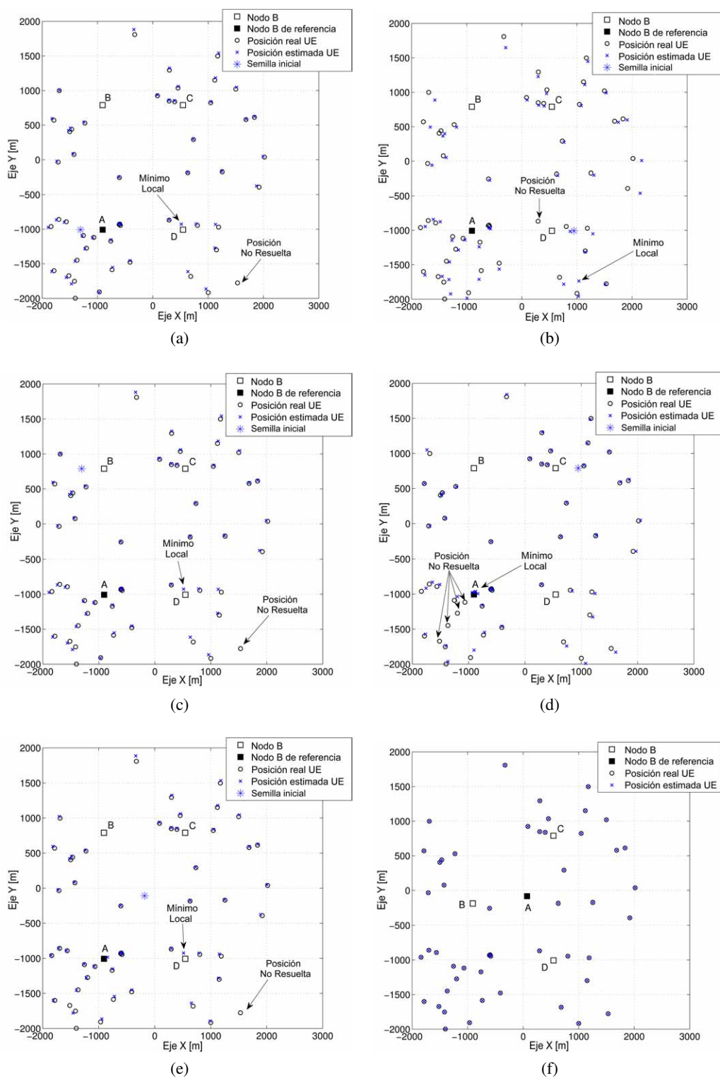
Figura 3.11: Escenarios con una configuración de sites en rectángulo e idénticas posiciones de los eventos en todos los casos. Los eventos son ideales y sintéticos, es decir, sin errores asociados. Los valores iniciales para el algoritmo de Levenberg-Marquardt fueron elegidos cerca de cualquiera de los sites involucrados en el escenario, tal y como se muestra en los casos (a) hasta (d); y en el centro de masas de los sites, tal y como indica (e). Todos ellos son comparados con la configuración en estrella recogida en (f), la cual ha empleado los mismos valores iniciales mencionados para la configuración rectangular. En el caso de la estrella, siempre se consigue exactamente la misma solución.
