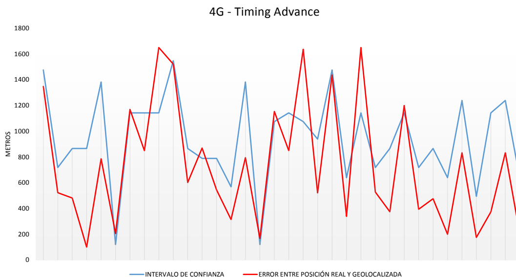
Figura 4.15: Comparativa entre el intervalo de confianza y el error real cometido por el método del timing advance, donde cada referencia del eje x es un evento geolocalizado.
