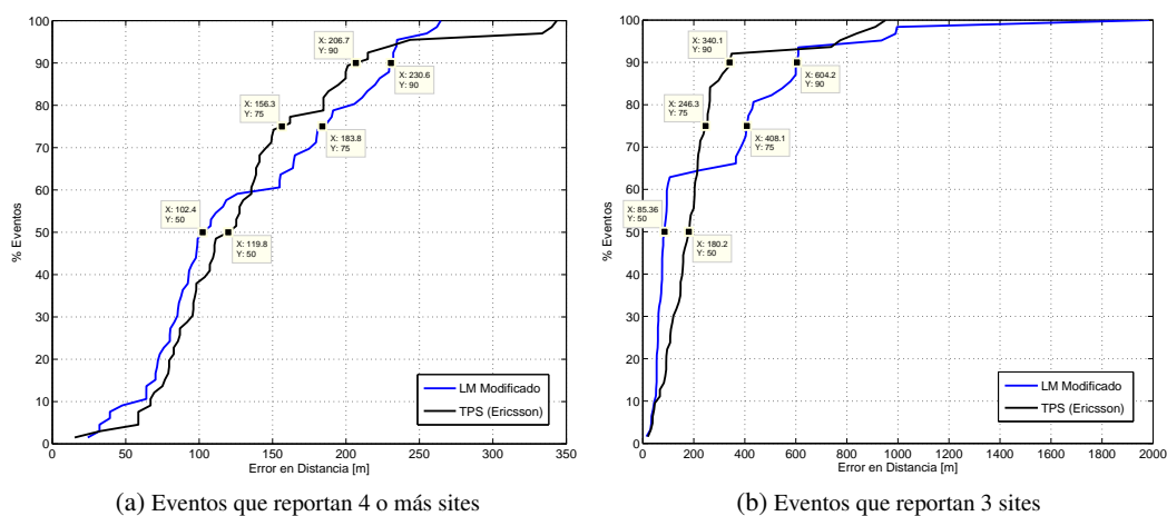
Figura 3.38: CDF del error de distancia correspondiente al cuarto ROP del set de datos de Europa. Se representa la comparativa de precisión obtenida en una región suburbana entre LM modificado y TPS. En primer lugar, se ilustra en (a) el error correspondiente a los eventos calculados directamente por la herramienta OTDOA, mientras que en (b) se representa el error de los eventos calculados posteriormente fijando las RTDs.
