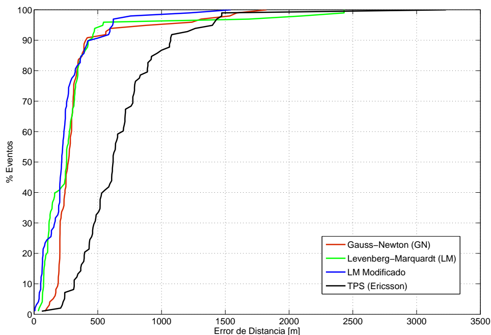
Figura 3.35: CDF del error de distancia correspondiente al primer ROP del set de datos de Europa en el caso de eventos que reportan solamente 3 sites. Para ello, se aprovechan los valores de sincronización entre sites obtenidos en la ejecución de la herramienta de geolocalización hiperbólica. Se representa la comparativa de precisión obtenida en una región suburbana entre GN, LM, LM modificado y TPS [30, 86].
