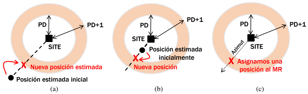
Figura 2.24: Uso del PD para refinar la posición del MR. Se muestran tres de las cuatro posibles situaciones, en concreto aquellas donde se lleva a cabo una acción sobre la posición del MR. (a) MR inicialmente en la parte exterior de la corona circular; (b) MR inicialmente en la parte interior de la corona circular; (c) MR no geolocalizado previamente.
