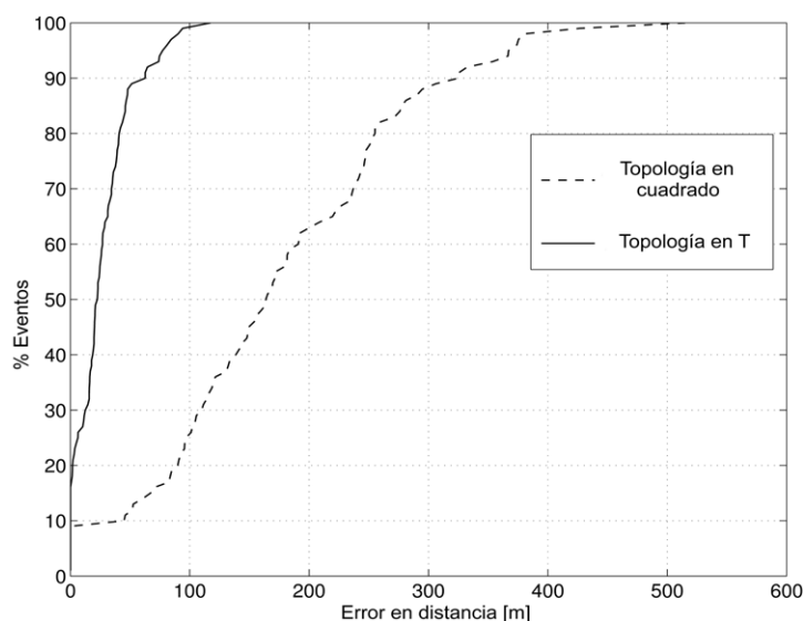
Figura 3.28: Distribución del error de geolocalización en un conjunto de escenarios ideales con topología en cuadrado y en T. La geometría en estrella no aparece representada, ya que en todas las simulaciones las estimaciones presentaban 0 metros de error [31].
