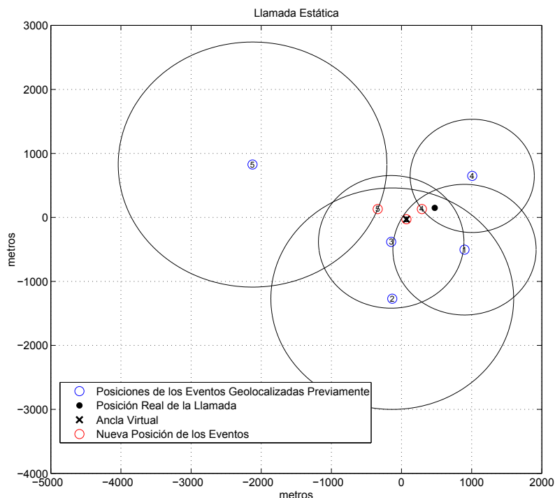
Figura 4.12: La imagen muestra una llamada estática simulada de la que se han geolocalizado cinco eventos. Cada evento representa el centro de la circunferencia que simboliza su intervalo de confianza al 95%. Entonces, el compresor fuerza la posición de los eventos 1, 2 y 3 hacia la posición del ancla virtual, ya que esta última cae dentro de las áreas de confianza de tales eventos. Por otro lado, los eventos 4 y 5 se quedan geolocalizados en el borde de sus intervalos de confianza.
