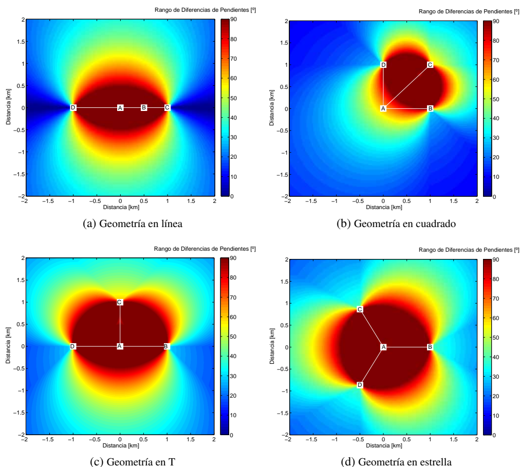
Figura 3.15: Rango de diferencias de pendientes evaluado para distribuciones de sites en: (a) línea recta, (b) cuadrado, (c) disposición de ‘T’, y (d) estrella. En todos los casos, el site ‘A’ es el site de referencia para que todas las medidas diferenciales sea tomadas con respecto a él.
