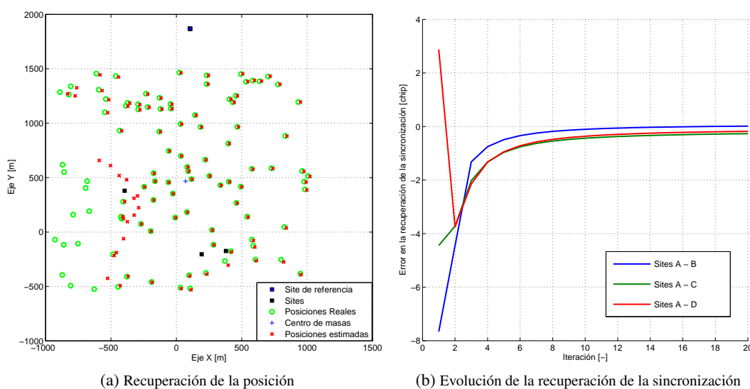
Figura 3.32: Escenario OTDOA sintético resuelto mediante Gauss-Newton. En (a) se representa la comparativa visual entre las posiciones reales y las estimadas. Por su parte, en (b) se ilustra la evolución de la recuperación de la sincronización a lo largo de las primeras 20 iteraciones del método numérico. Se observa que aproximadamente a partir de la iteración 10, el error en las estimaciones de las RTDs se estabiliza sin que se llegue a alcanzar por completo los valores buscados.
