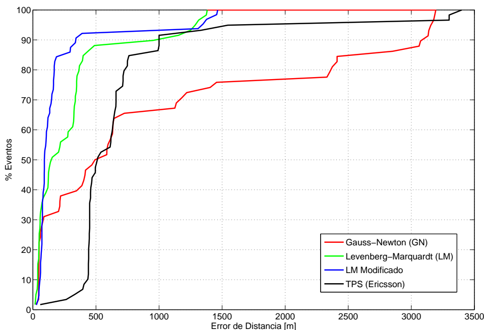
Figura 3.34: CDF del error de distancia correspondiente al primer ROP del set de datos de Europa. Se representa la comparativa de precisión obtenida en una región suburbana entre GN, LM, LM modificado y TPS [30, 86].
