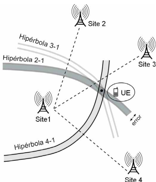
Figura 3.3: Ejemplo de multilateración hiperbólica en un escenario conformado por 4 sites. Se han representado las tres hipérbolas que se generan tomando el site 1 como referencia. Asimismo, el grosor de las hipérbolas es debido a posibles errores en las medidas causados, por ejemplo, por el multitrayecto o el redondeo.
