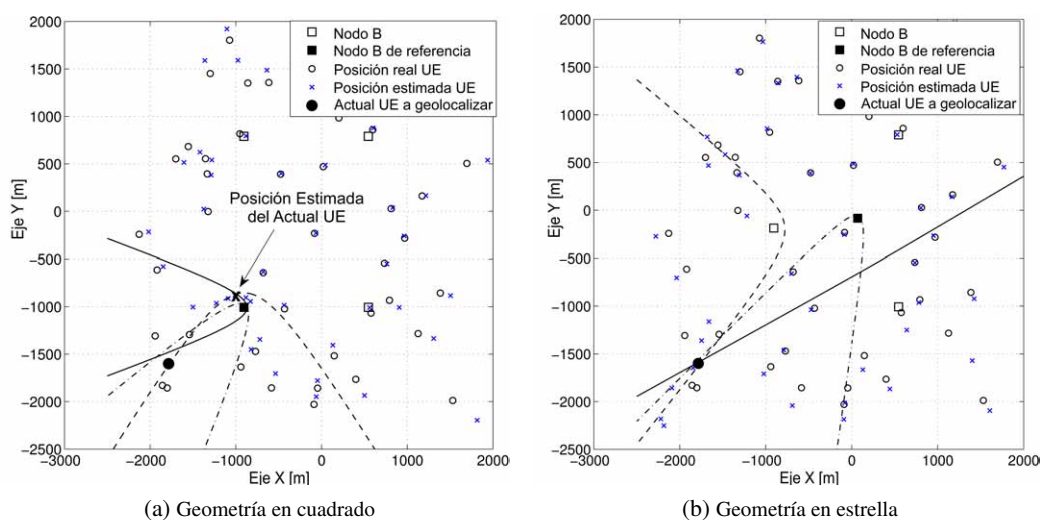
Figura 3.12: Escenarios con eventos sintéticos a los que se le ha añadido el error por redondeo del parámetro T_M a todas las medidas. Por otro lado, (a) muestra una configuración de 4 sites en rectángulo y (b) en estrella. Las tres hipérbolas dibujadas se refieren a un UE particular representado como un círculo grande negro. Como resultado, el mínimo local detectado en la configuración rectangular es evitado al emplear la geometría en estrella. Asimismo, la posición estimada para el UE particular bajo análisis es resaltada con una 'X' en negrita para el caso (a).
