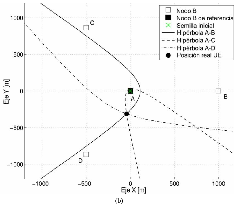
Figura 3.19: Aspecto de las hipérbolas en un escenario con geometría en estrella cuando los puntos a geolocalizar están en áreas de alto rango de diferencias de pendientes.
