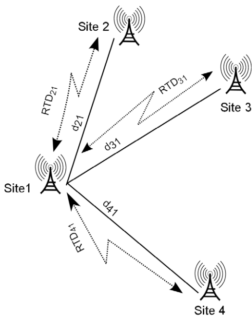
Figura 3.4: Escenario básico de 4 sites, donde se resaltan las relaciones entre el site de referencia (site 1) y el resto. Por un lado, los ejes focales corresponden a las distancias entre los sites ( d_{21}, d_{31}, d_{41} ). Por otro lado, las RTDs relacionan las diferencias de sincronización.
