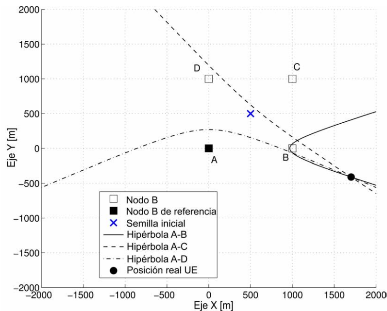
Figura 3.22: Caso 2: Aspecto de las hipérbolas en un escenario con geometría en cuadrado cuando los puntos a geolocalizar están en áreas de bajo rango de diferencias de pendientes —ver Fig. 3.15(b)—.
