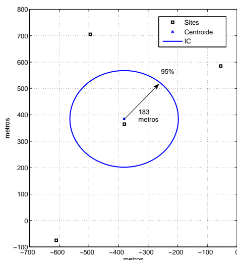
Figura 4.2: Se muestra un ejemplo real del intervalo de confianza al 95 % calculado para el método del centroide. La posición estimada del evento es la cruz azul (centroide), mientras que la circunferencia es el área de incertidumbre, la cual tiene un radio de 183 metros.
