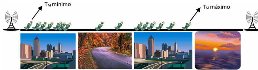
Figura 3.31: Ejemplo de mala estimación inicial de la RTD. La zona más cercana al site de la derecha está ubicada en un lago, donde, como es evidente, es difícil encontrar algún UE reportado. Por tanto, cuando se calcula el valor medio de la banda con los UEs extraídos de los MRs, el valor hallado saldrá bastante desplazado a la izquierda de su posición real, ya que el T_M máximo está muy distorsionado con respecto al valor esperado. Sin duda, esta técnica para extraer semillas iniciales de las RTDs es muy dependiente de la situación geográfica debido a que podemos encontrar edificios y zonas despobladas entre dos sites.
