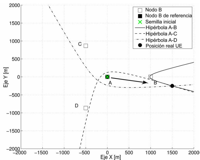
Figura 3.25: Caso 1: Aspecto de las hipérbolas en un escenario con geometría en estrella cuando los puntos a geolocalizar están en áreas de bajo rango de diferencias de pendientes —ver Fig.3.15(d)—.
