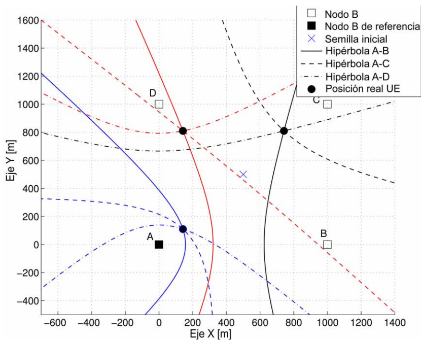
Figura 3.18: Aspecto de las hipérbolas en un escenario con geometría en cuadrado cuando los puntos a geolocalizar están dentro del polígono formado por los cuatro sites.
