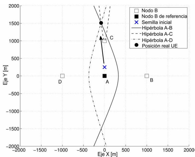
Figura 3.24: Caso 2: Aspecto de las hipérbolas en un escenario con geometría en T cuando los puntos a geolocalizar están en áreas de bajo rango de diferencias de pendientes —ver Fig.3.15(c)—.
