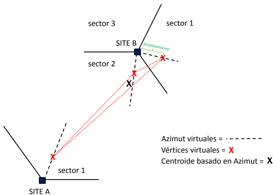
Figura 2.21: Procedimiento de geolocalización basado en azimut.
