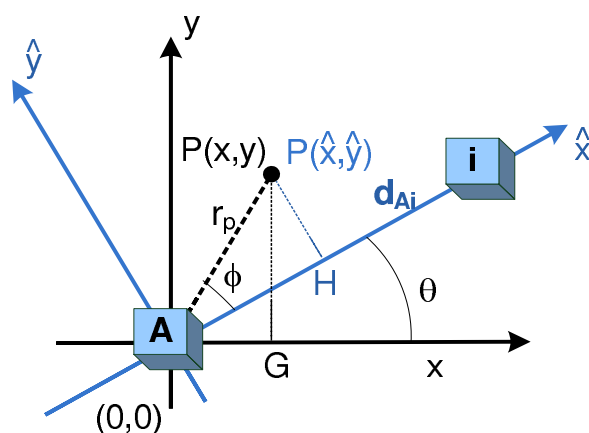
Figura 3.13: Rotación de los ejes de coordenadas x e y .
