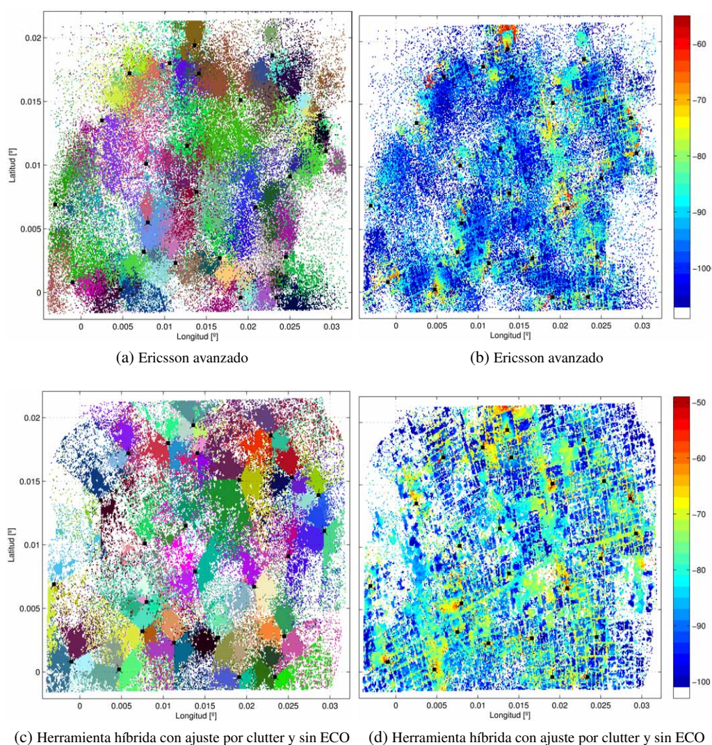
Figura 2.40: Rásters best server (izquierda) y nivel de señal en dBms (derecha) en Asia.
