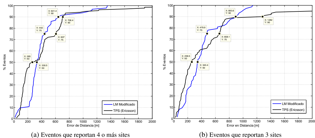
Figura 3.37: CDF del error de distancia correspondiente al tercer ROP del set de datos de Europa. Se representa la comparativa de precisión obtenida en una región suburbana entre LM modificado y TPS. En primer lugar, se ilustra en (a) el error correspondiente a los eventos calculados directamente por la herramienta OTDOA, mientras que en (b) se representa el error de los eventos calculados posteriormente fijando las RTDs.
