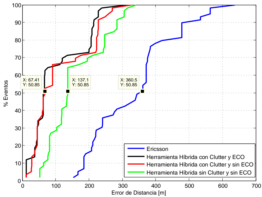
Figura 2.35: CDFs del error de distancia punto a punto para el escenario de Málaga. Se comparan cuatro alternativas, señalando como punto clave el percentil 50.
