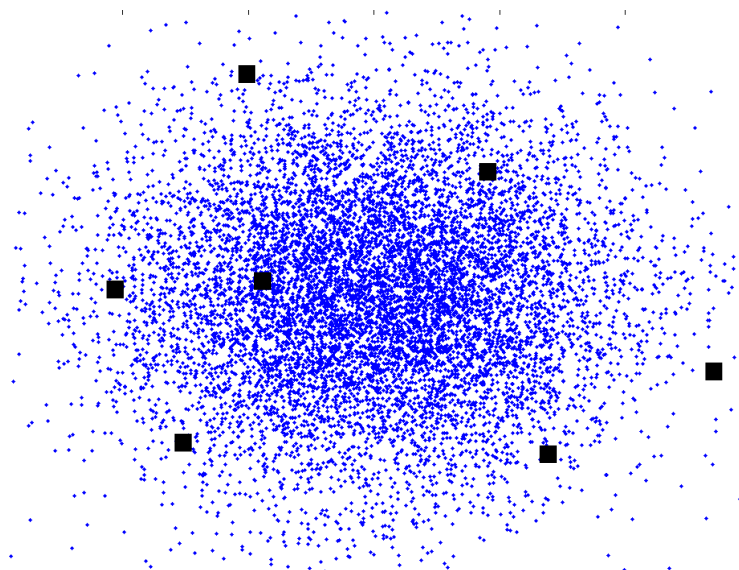
Figura 4.7: Escenario sintético compuesto de 100,000 eventos virtuales y 7 sites sobre el que se aplica la técnica de multilateración.
