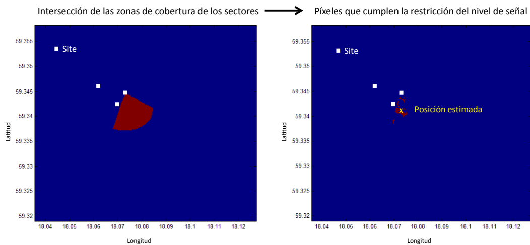
Figura 2.22: Geolocalización basada en el nivel de señal. Los píxeles rojos representan los píxeles candidatos o válidos. La primera selección se realiza mediante la intersección de zonas de cobertura (figura de la izquierda), y la segunda a través de la discrepancia de nivel de señal medido y estimado (figura de la derecha). Después, la posición estimada viene dada por la posición media de los píxeles subsistentes.
