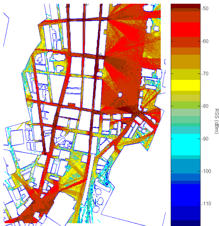
Figura 2.8: Técnica de posicionamiento RSS usando huellas de potencia [47].
