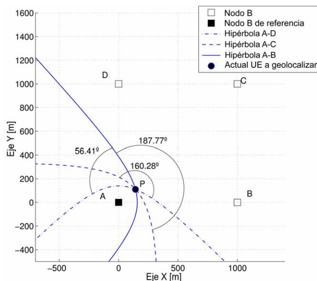
Figura 3.14: Diferencias de pendientes de tres hipérbolas en un determinado punto P para un escenario con topología rectangular.
