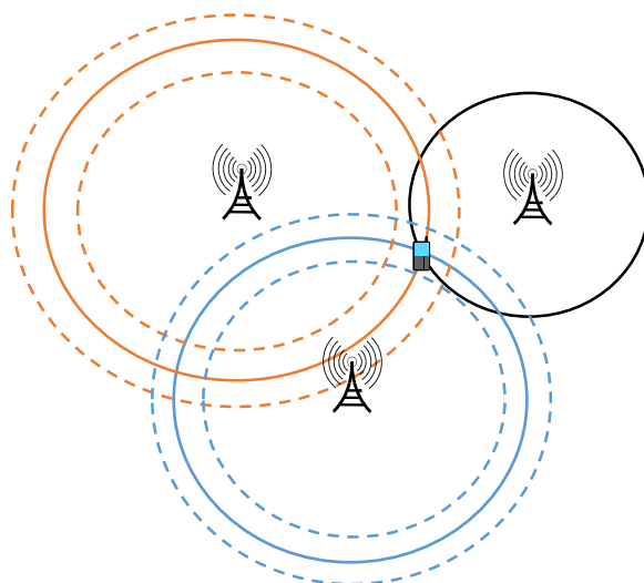
Figura 2.3: Técnica de posicionamiento TOA usando la trilateración. Las circunferencias con línea continua están asociadas a las medidas ideales, dando como resultado la posición exacta del UE. Por su parte, las circunferencias discontinuas serían consecuencia de errores en los niveles de señal medidas generando un área de incertidumbre. El Nodo B que hace de centro a la circunferencia negra no tiene circunferencias con error para una mayor claridad en el dibujo.
