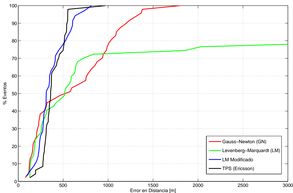
Figura 3.40: CDF del error de distancia correspondiente al set de datos de Norteamérica en el caso de eventos que reportan solamente 3 sites. Para ello, se aprovechan los valores de sincronización entre sites obtenidos en la ejecución de la herramienta de geolocalización hiperbólica. Se representa la comparativa de precisión obtenida en una región suburbana entre GN, LM, LM modificado y TPS [30][II].
