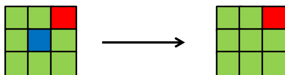
Figura 2.28: Interpolación de píxeles, donde si, al menos, 7 de los 8 píxeles adyacentes tienen un mismo valor, el píxel central pasa a tomar ese valor.
