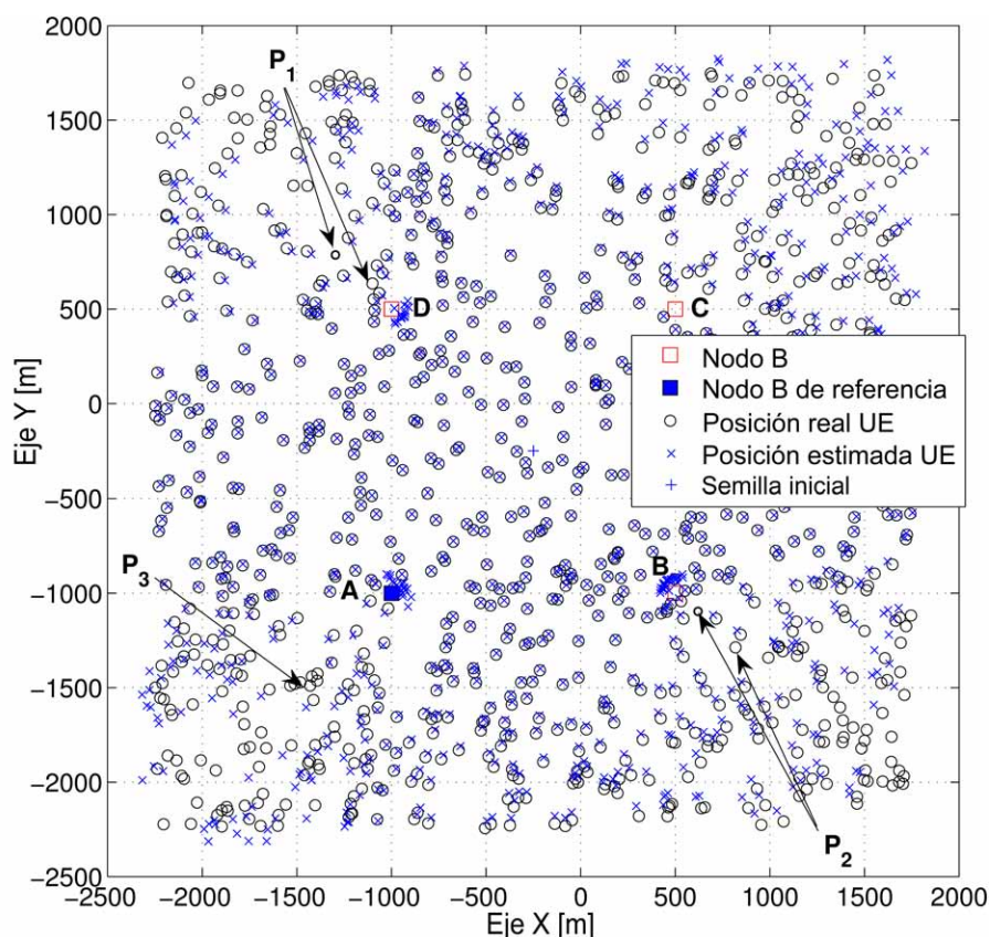
Figura 3.16: Escenario de 1000 eventos reportando cuatro sites dispuestos en cuadrado.
