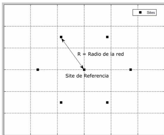
Figura 4.6: Escenario hexagonal de referencia para hallar el IC de la multilateración hiperbólica. El site de referencia se sitúa en el centro, y el tamaño de la red queda definido por el parámetro R .
