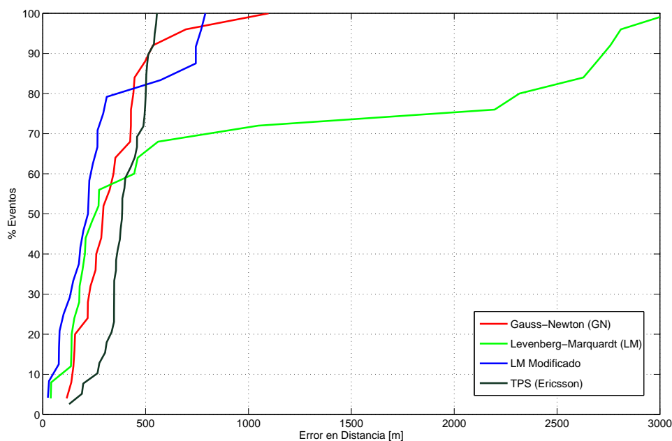
Figura 3.39: CDF del error de distancia correspondiente al set de datos de Norteamérica. Se representa la comparativa de precisión obtenida en una región suburbana entre GN, LM, LM modificado y TPS [30, 86].
