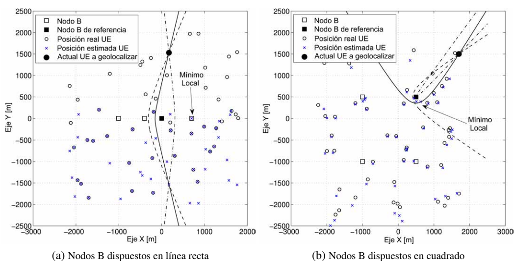
Figura 3.7: Ejemplos de malas geometrías: (a) La geometría en línea recta manifiesta una ambigüedad irresoluble en la estimación de las posiciones de los UEs. Además, mínimos locales son detectados en el extremo de los ejes focales. (b) Sites colocados en cuadrado con presencia de mínimos locales. Para el actual UE a geolocalizar, en la intersección de las 3 hipérbolas, el algoritmo iterativo falla porque se forma un mínimo local cerca del Nodo B de referencia. Ahí, se produce la intersección de dos hipérbolas, muy cerca en el espacio a la tercera hipérbola, por lo que la función de coste llega a ser muy pequeña.
