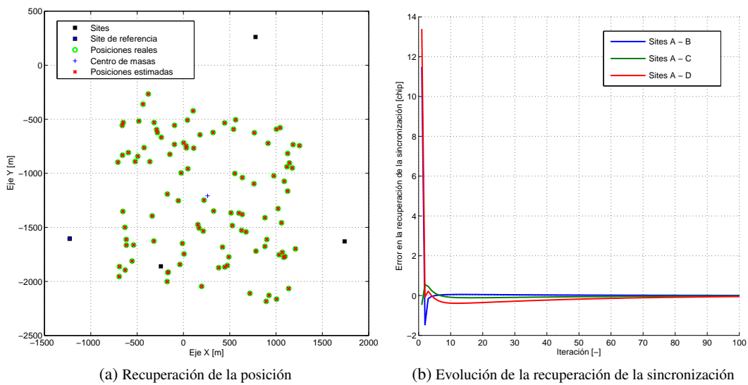
Figura 3.33: Escenario OTDOA sintético resuelto mediante Levenberg-Marquardt. En (a) se representa la comparativa visual entre las posiciones reales y las estimadas al final de la ejecución del algoritmo. Por su parte, en (b) se ilustra la evolución de la recuperación de la sincronización a lo largo de las primeras 100 iteraciones del método numérico. Se observa que finalmente las estimaciones de las RTDs acaban convergiendo a los valores deseados.
