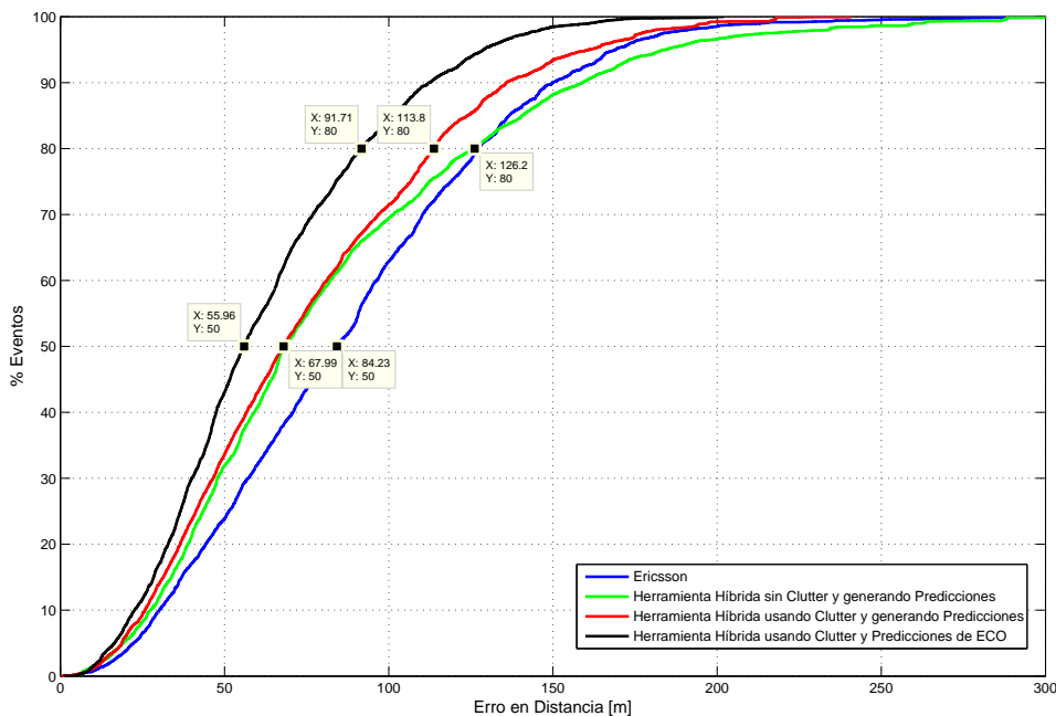
Figura 2.29: CDFs del error de distancia punto a punto para el escenario del norte de Europa. Se comparan cuatro alternativas, señalando como puntos clave el percentil 50 y el percentil 80.
