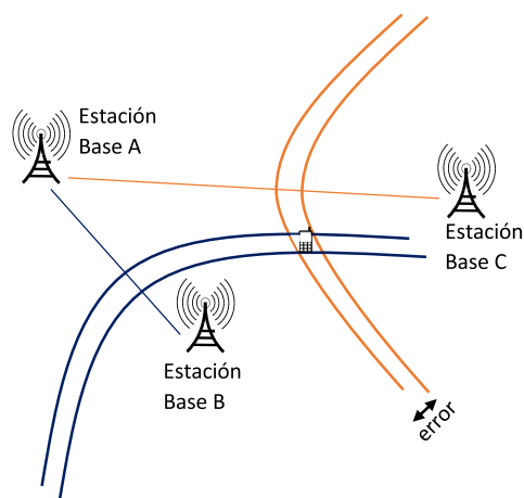
Figura 2.4: Técnica de posicionamiento TDOA. La hipérbola azul corresponde a la formada por los focos A-B, mientras que la naranja está relacionada a los focos A-C. Además, las hipérbolas no se han trazado con una sola línea, sino que se las ha dibujado con cierto grosor para representar el efecto de posibles errores como el multipath .
