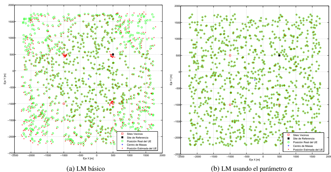
Figura 3.6: Simulación de un escenario con los sites en geometría de cuadrado y 1000 UEs distribuidos por el espacio de alrededor. En la izquierda, el uso de LM básico hace que muchos eventos acaben erróneamente localizados en mínimos locales generados en las inmediaciones de los sites. En la derecha, el parámetro \alpha permite "saltar" esos mínimos locales logrando que la localización de todos los eventos sean perfectamente estimada.
