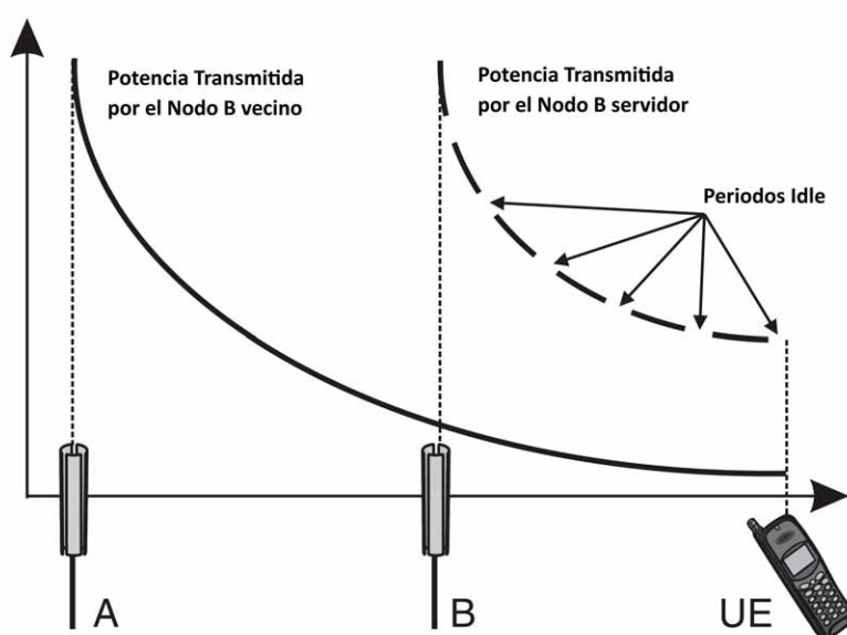
Figura 3.1: Funcionamiento de los periodos inactivos ( idle periods ) en OTDOA. El Nodo B llamado "B" ejerce como servidor enmascarando la señal del Nodo B llamado "A", teniendo en cuenta que el eje vertical representa la potencia de señal. Entonces, se aprovecha los periodos de inactividad de "B" para recibir a "A" [7].
