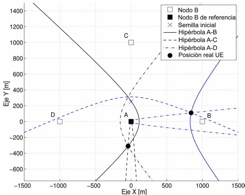
Figura 3.20: Aspecto de las hipérbolas en un escenario con geometría en T cuando los puntos a geolocalizar están en áreas de alto rango de diferencias de pendientes.
