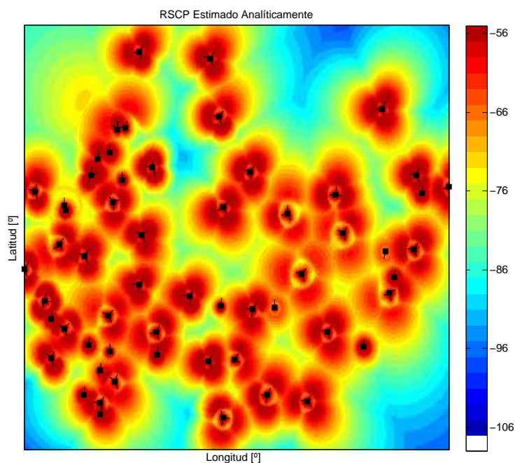
Figura 2.18: RSCP [dBm] estimado en una red real.
