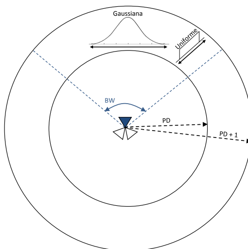
Figura 4.3: En la imagen se representa un site tri-sectorial, resaltando uno de los sectores junto a su BW. Un evento que ha medido un valor de PD con respecto a ese sector debe quedar localizado en la corona circular comprendida entre PD y PD+1. La posición dentro de esa zona delimitada quedará determinada angularmente por una distribución de probabilidad Gaussiana y, radialmente, por una uniforme.
