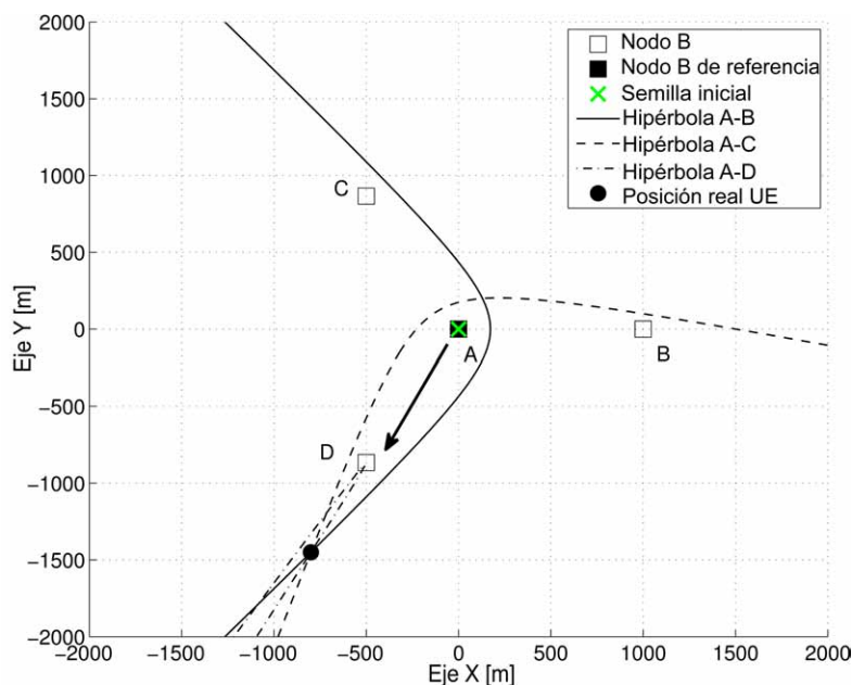
Figura 3.27: Caso 3: Aspecto de las hipérbolas en un escenario con geometría en estrella cuando los puntos a geolocalizar están en áreas de bajo rango de diferencias de pendientes —ver Fig.3.15(d)—.
