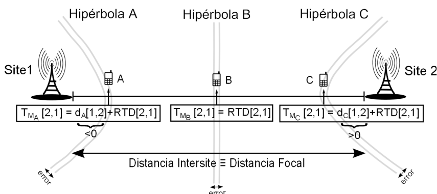
Figura 3.29: Representación del concepto de banda como el rango en el que pueden acotarse los valores del parámetro T_M . Tres UEs denominados A , B y C están colocados en tres posiciones distintas a lo largo del eje focal, que es la línea que separa los sites 1 y 2. T_{M_i} , i \in A, B, C representa el valor ideal medido por cada UE, donde se aprecia que la RTD[2, 1] es constante en las tres medidas. Asimismo, la diferencia de distancia toma valores negativos ( d_A ) en la parte derecha (hipérbolas que se cierran en torno al site 1) y valores positivos ( d_C ) en la parte izquierda (hipérbolas que se cierran en torno al site 2).
