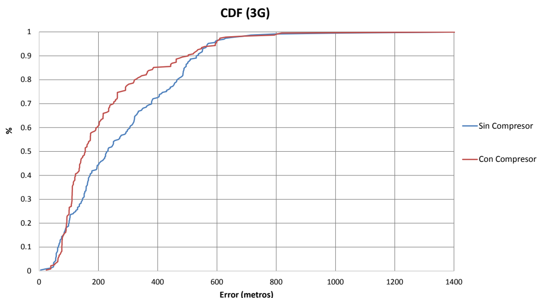
Figura 4.19: CDFs del error cometido al geolocalizar antes y después de aplicar el compresor en una red 3G [I].
