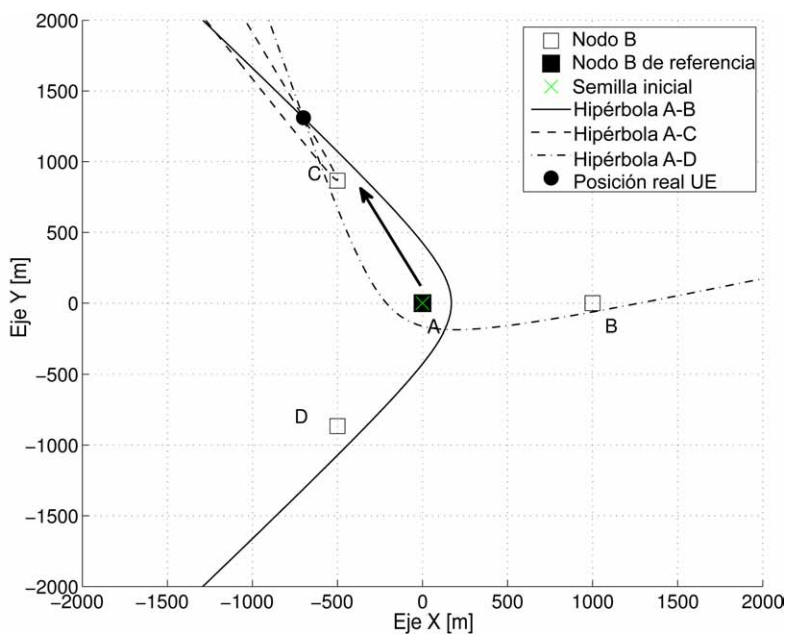
Figura 3.26: Caso 2: Aspecto de las hipérbolas en un escenario con geometría en estrella cuando los puntos a geolocalizar están en áreas de bajo rango de diferencias de pendientes —ver Fig.3.15(d)—.
