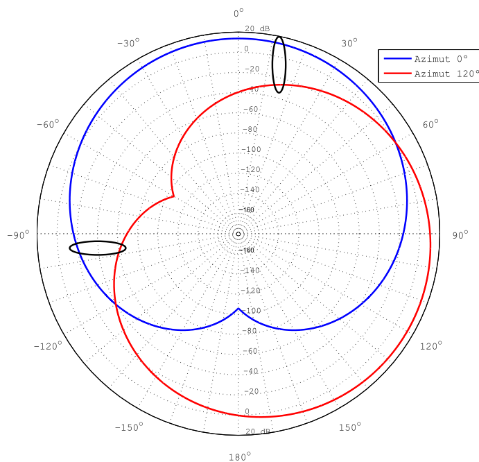
Figura 4.8: Aplicación del método AOA cuando se emplean medidas de sectores del mismo site. Se han representado los diagramas de radiación de dos sectores cuyos azimuts apuntan a 0^\circ (azul) y 120^\circ (rojo), respectivamente. Además, se ha señalado con elipses negras un ejemplo que representa que siempre hay dos ángulos para los que se cumple que la diferencia de ganancia entre los sectores es igual, en este caso unos 40 dB.
