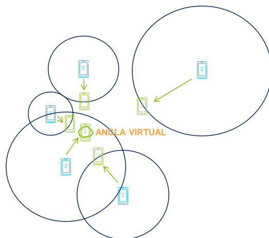
Figura 4.11: Funcionamiento teórico del compresor con cinco eventos (móviles azules) que se hallan en el centro de las circunferencias que representan sus correspondientes intervalos de confianza al 95%. Tras aplicar el compresor, las nuevas posiciones de los eventos (móviles verdes) se agrupan en torno al ancla virtual según los criterios definidos previamente. De hecho, uno de los eventos termina desplazado justamente en la posición del ancla virtual.
