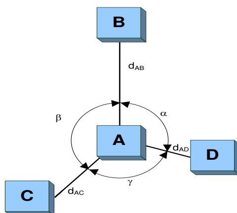
Figura 3.9: Sites situados en una geometría en estrella formada por cuatro sites nombrados 'A', 'B', 'C' y 'D', siendo 'A' el site de referencia. Los ángulos entre dos de estos sites ( \alpha , \beta , \gamma ) deben estar entre 100^\circ y 140^\circ , esto es, 1.75 y 2.44 rads. Por otro lado, la distancia entre el site más lejano y el más cercano con respecto al site de referencia no debería exceder la proporción 3:1.
