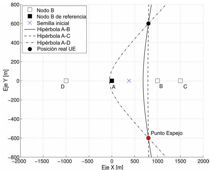
Figura 3.17: Aspecto de las hipérbolas en un escenario con geometría en línea. También se representa el punto espejo derivado de este tipo de topologías.
