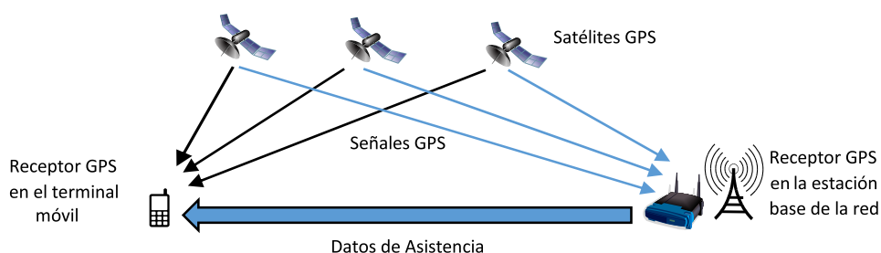
Figura 2.7: Técnica de posicionamiento A-GPS.
