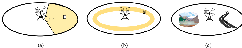
Figura 2.1: Posibles mejoras sobre el método básico de posicionamiento conocido como Cell ID. (a) Usar antenas sectoriales; (b) usar el RTT; (c) aprovechar la información del terreno.
