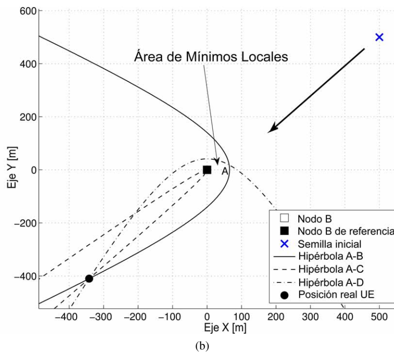
Figura 3.21: Caso 1: Aspecto de las hipérbolas en un escenario con geometría en cuadrado cuando los puntos a geolocalizar están en áreas de bajo rango de diferencias de pendientes —ver Fig.3.15(b)—. Además, en (b) se muestra una ampliación de (a) para una mejor apreciación de las hipérbolas.
