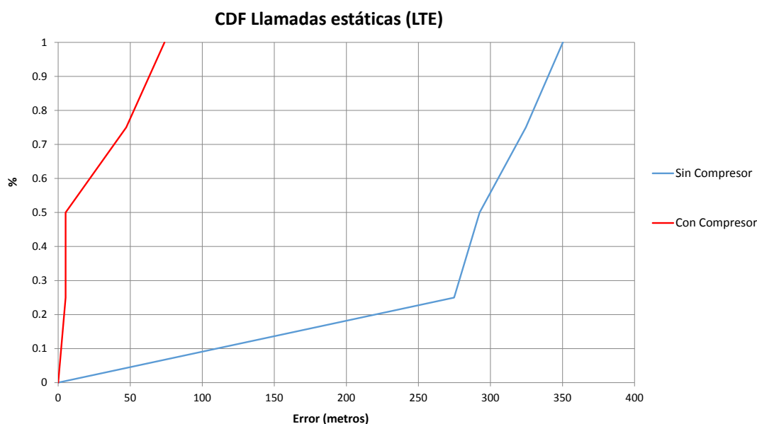
Figura 4.20: CDFs del error cometido al geolocalizar antes y después de aplicar el compresor sobre llamadas estáticas en una red LTE [I].
