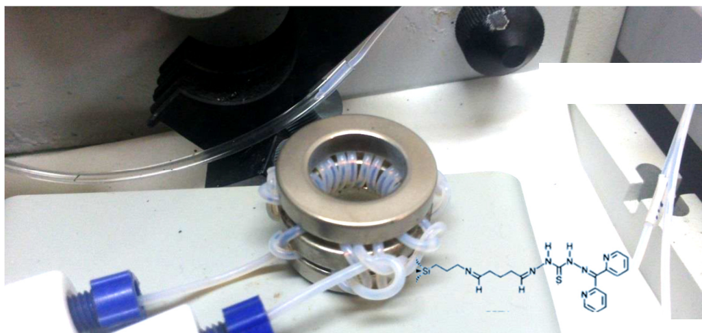
DPTH-MNPs
