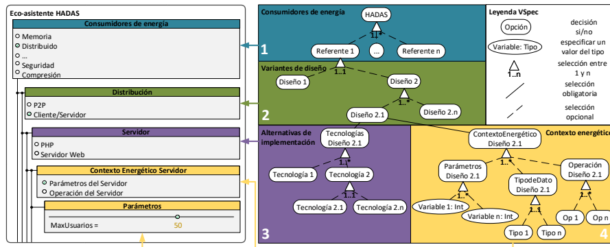
Figura 2. Estructura por niveles de la variabilidad del árbol y del formulario
