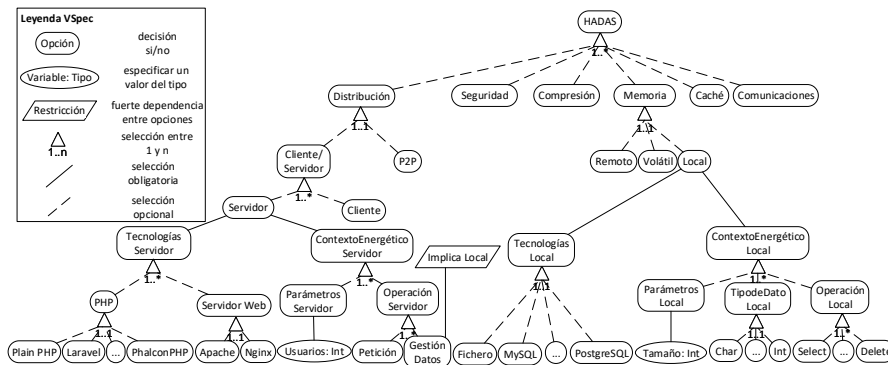
Figura 3. Caso de estudio de una aplicación web
