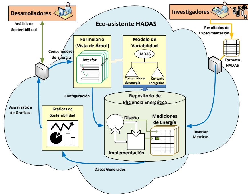
Figura 1. Visión general del eco-asistente HADAS
