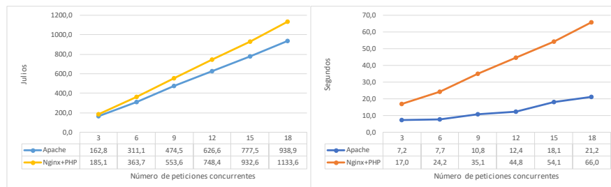
Figura 4. Consumo y tiempo de ejecución de Apache y Nginx, junto a PHP
