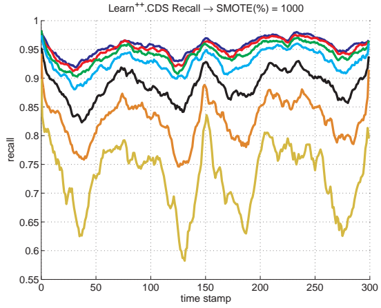
(d) SMOTE(%)=1000
