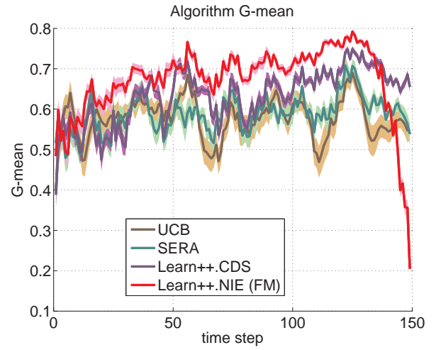
(d) G-mean
