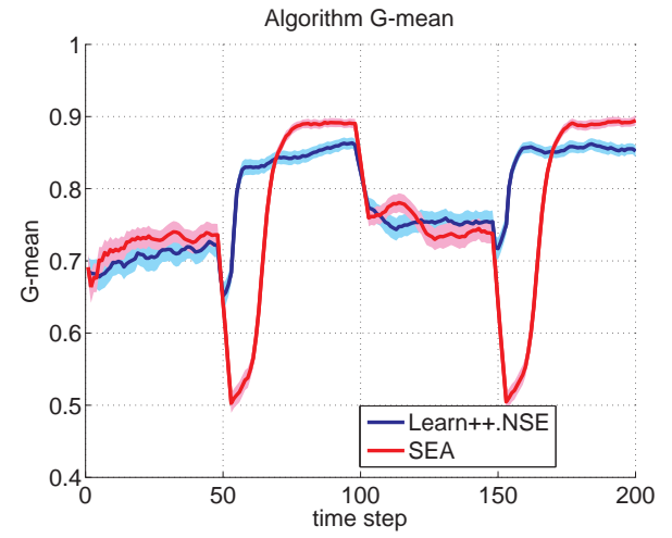
(d) G-mean
