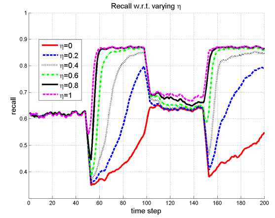
(d) Recall
