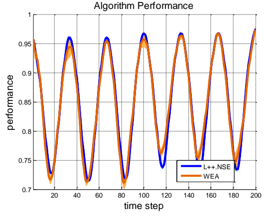
(b) Bias=1
