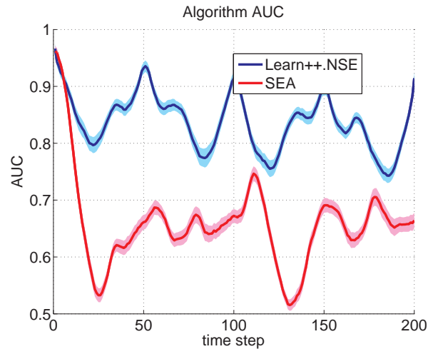
(h) AUC
