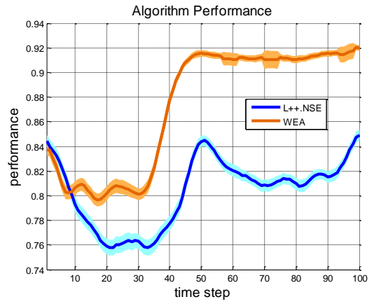
(d) Bias=5
