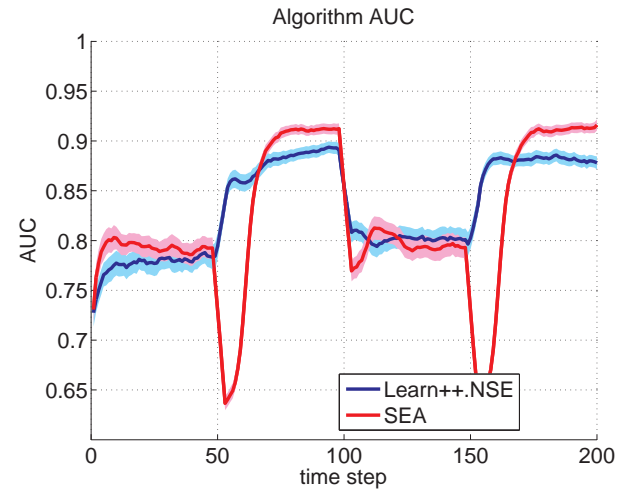
(b) AUC
