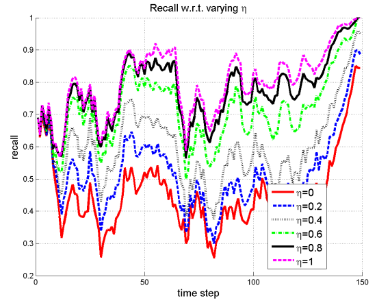
(d) Recall
