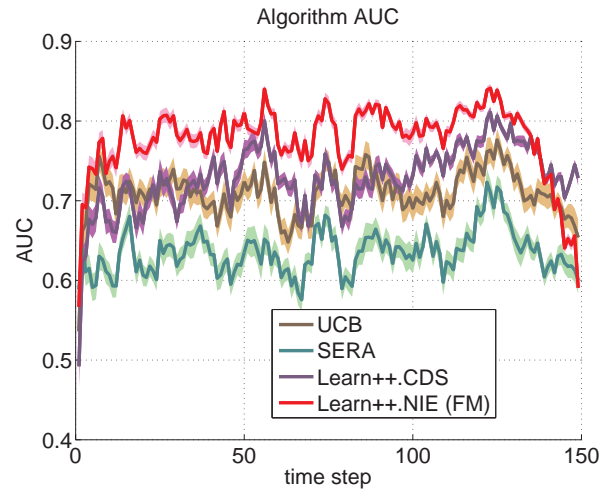
(b) AUC
