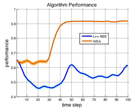
(f) Bias=10
