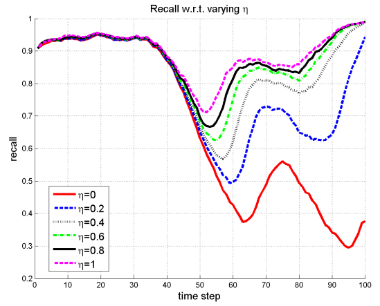
(d) Recall
