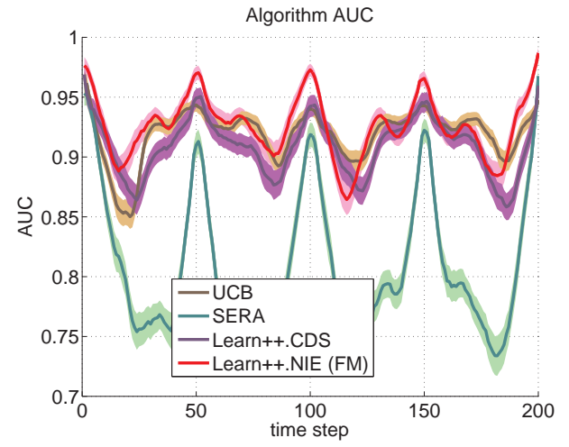
(b) AUC
