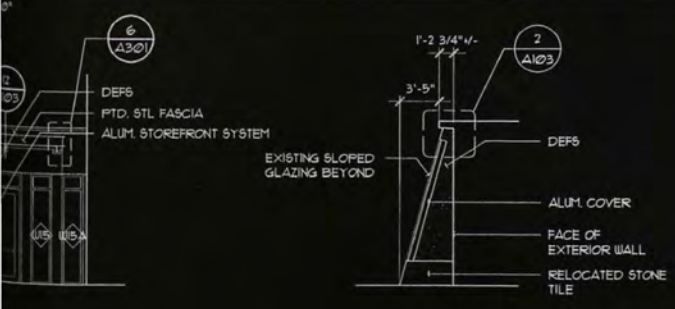
Elevation SCALE: 1/8"=1'-0"
