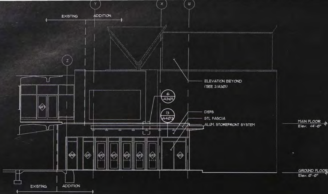
1 Elevation A301 SCALE: 1/8"=1'-0"
