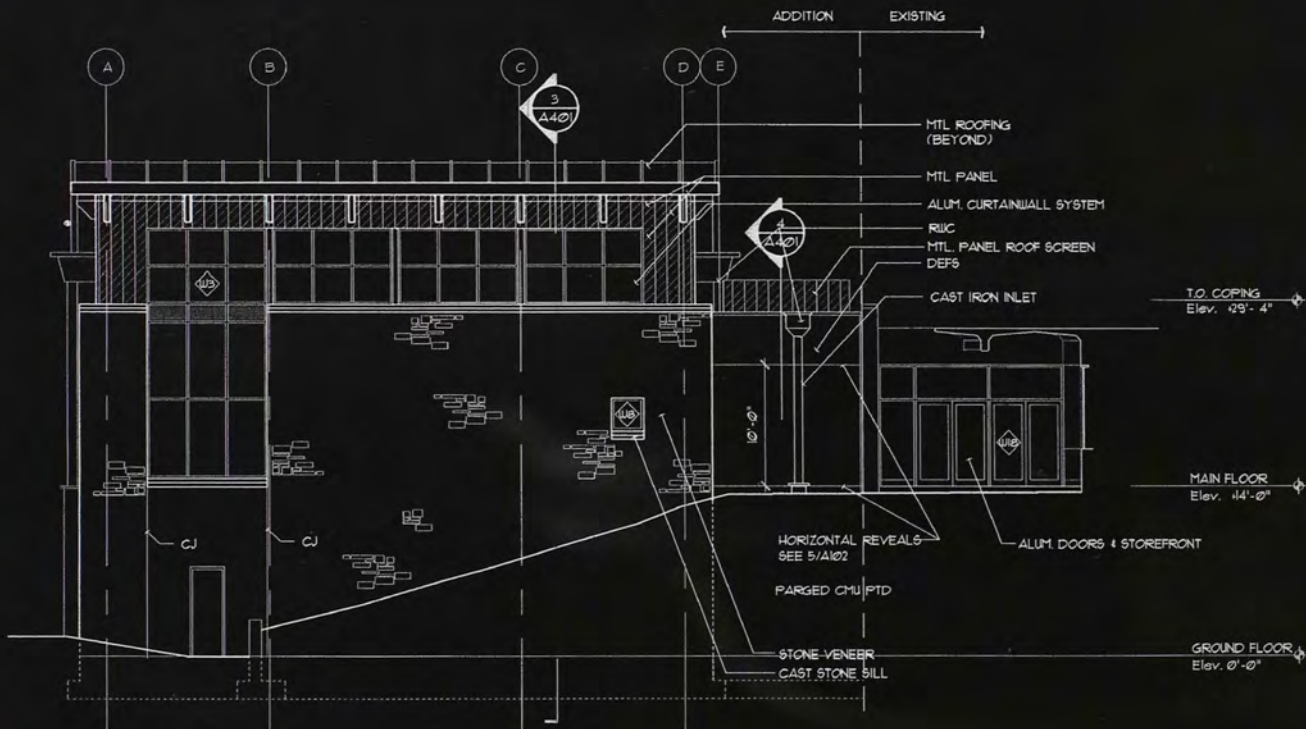
3 Elevation A301 SCALE: 1/8"=1'-0"
