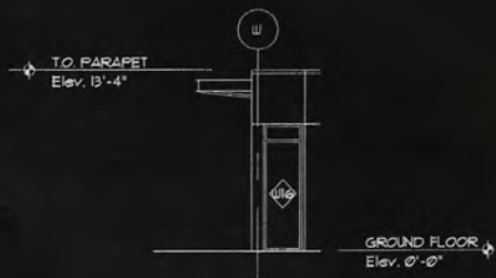
3 Elevation A301 SCALE: 1/8"=1'-0"
